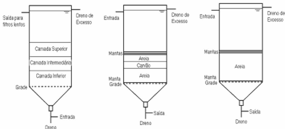
FIGURA 1. Esquema construtivo do pré-filtro e dos dois filtros lentos. Constructive scheme of the pre-filter and two slow sand filters.
