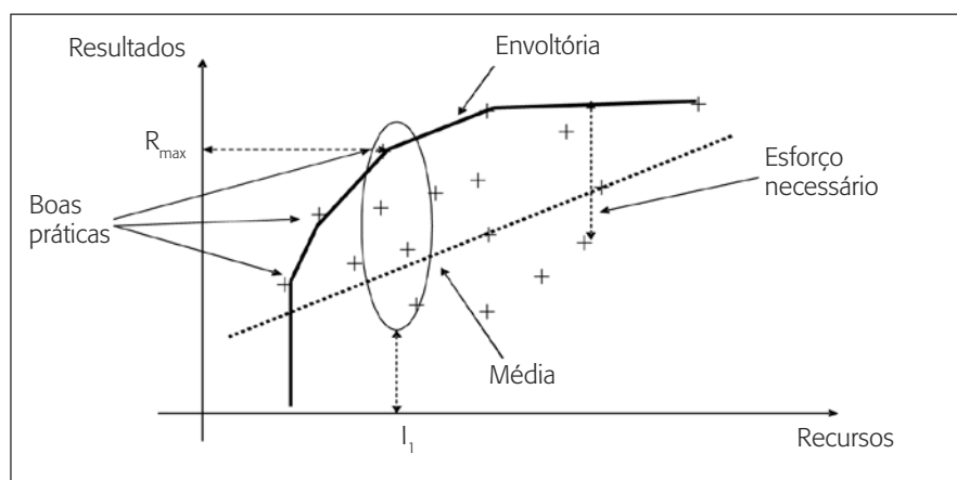
Figura 1 Esquema geral da análise envoltória de dados
