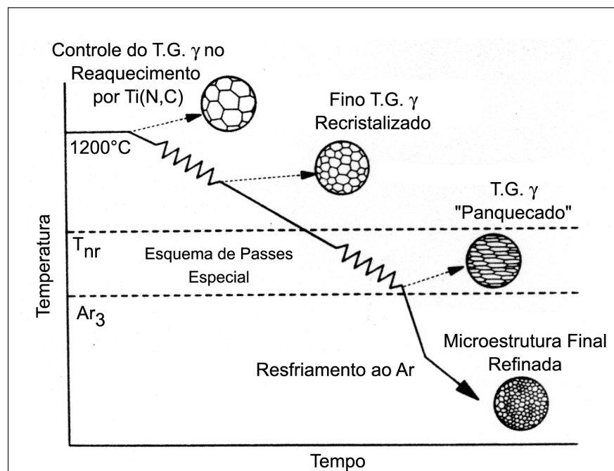
Figura 2 - Esquema da laminação controlada empregado no processamento de aços HSLA-80 e ULCB [Wilson, 1988].
