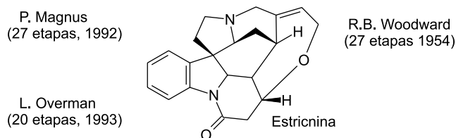
Figura 1. Algumas sínteses da estricnina
