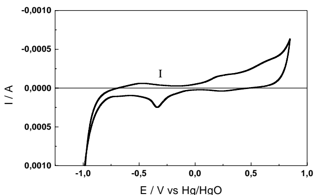
Figura 1. Voltamograma cíclico para o Pd policristalino, em solução de NaOH 1M a 22°C ( v = 0,05 \text{ V.s}^{-1} ).
