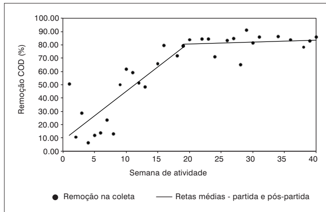
Figura 3 – Remoção dos valores de carbono orgânico (COD) dissolvido do efluente dos filtros anaeróbios em relação ao esgoto bruto durante o período do experimento.
