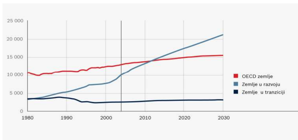
Графикон 4: Пораст емисије угљен-диоксида у свету 680
