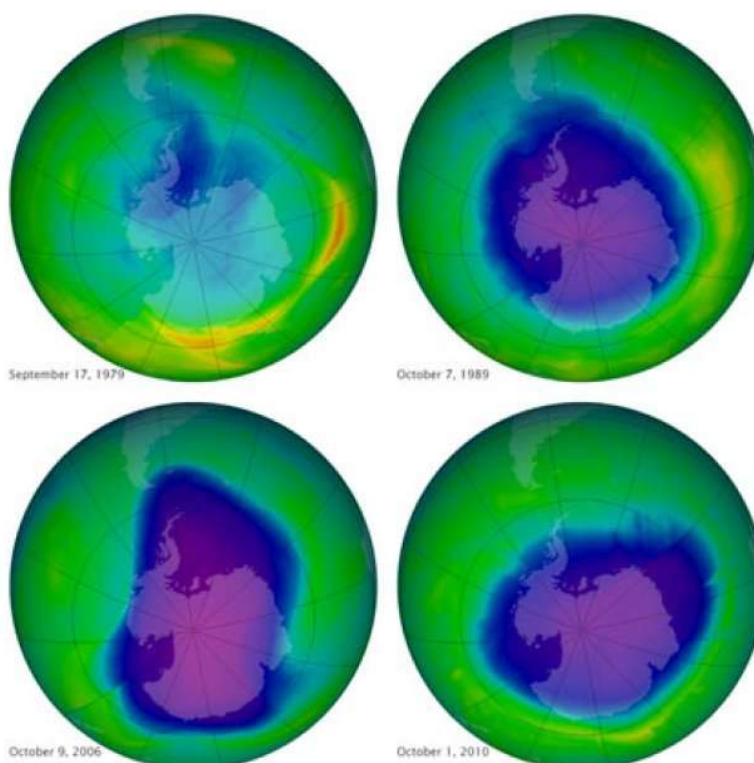
Слика 4: Озонска рупа изнад Антарктика (1979., 1989., 2006. и 2010. године) 666
