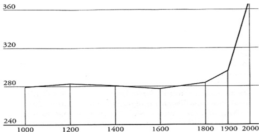
Графикон 3: Концентрација угљен диоксида у атмосфери (ppm) 677
