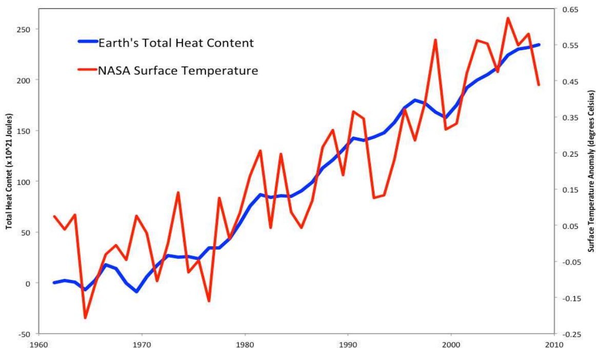
Графикон 2: Пораст укупне количине топлоте и температуре на глобалном нивоу од 1960-2010 673
