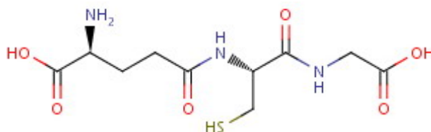
Slika 6. Struktura GSH
