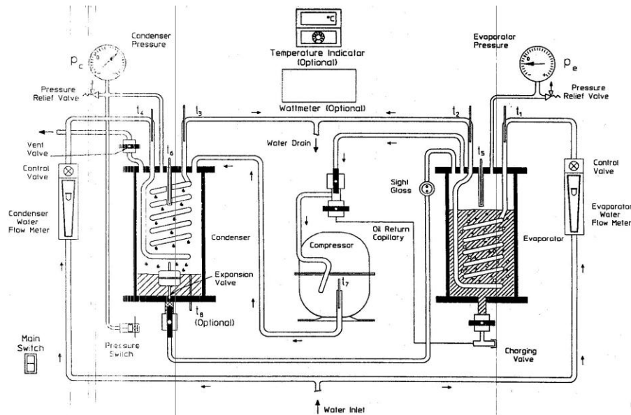
Gambar 2. Mesin Refreigerasi R 633
