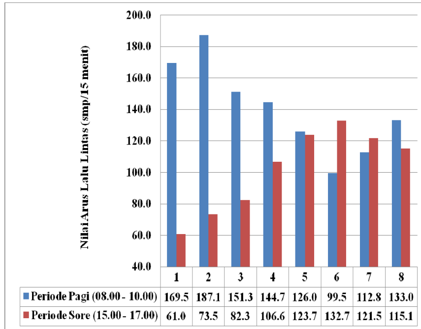
Gambar 5. Nilai Arus Lalu lintas Jl. Datu Pamusu pada Periode Jam Puncak Pagi dan Sore Hari
