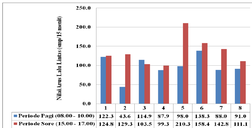
Gambar 3. Nilai Arus Lalu lintas Jl. Mangga pada Periode Jam Puncak Pagi dan Sore Hari
