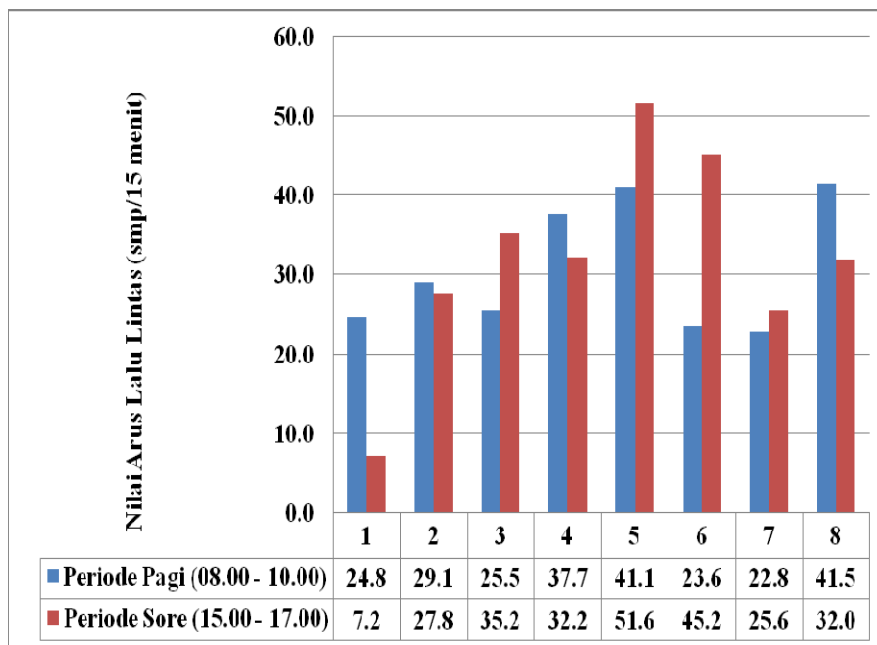
Gambar 6. Nilai Arus Lalu lintas Jl. S. Moutong pada Periode Jam Puncak Pagi dan Sore Hari
