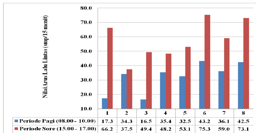
Gambar 4. Nilai Arus Lalu lintas Jl. S. Sausu pada Periode Jam Puncak Pagi dan Sore Hari
