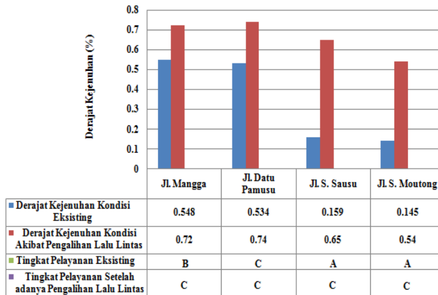
Gambar 7. Rekapitulasi Tingkat Pelayanan Ruas Ruas Jalan Lokasi Studi Setelah Pengalihan Arus Lalu lintas Jl. Sis Aljufri
