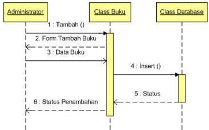
Gambar 3. Sequence Diagram Tambah Buku
