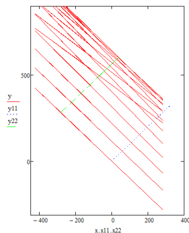
Рис.5. Горизонтальна проєкція поверхні полиці культурного типу
