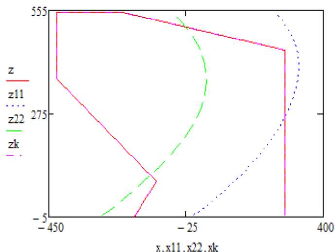
Рис. 3. Фронтальна проєкція лобового контуру та напрямних кривих
