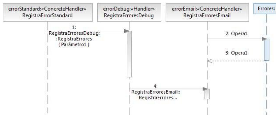
Fig. 5. Ejemplo 2 Diagrama de secuencia generador de logs
