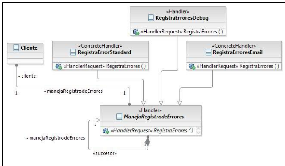
Fig. 3. Diagrama de clases generador de logs
