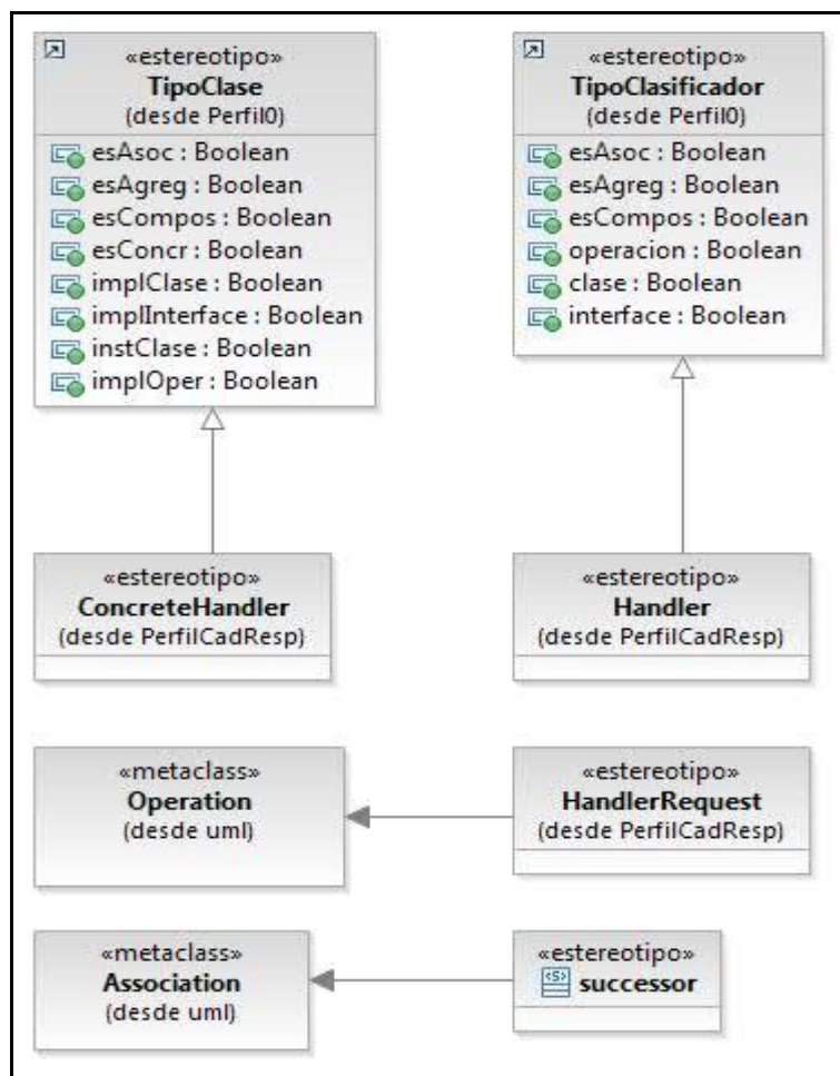
Fig. 1. Perfil de Patron Cadena de Responsabilidad
