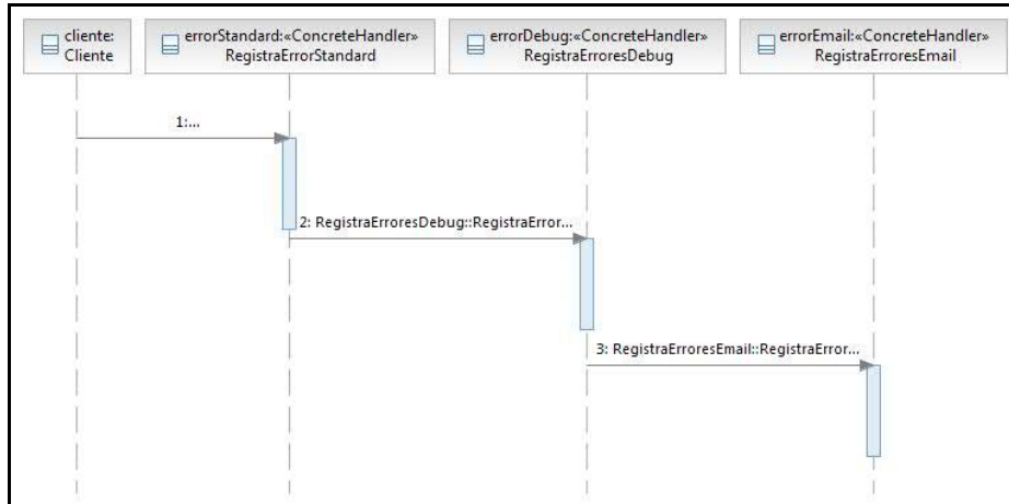
Fig. 4. Ejemplo 1 Diagrama de secuencia generador de logs
