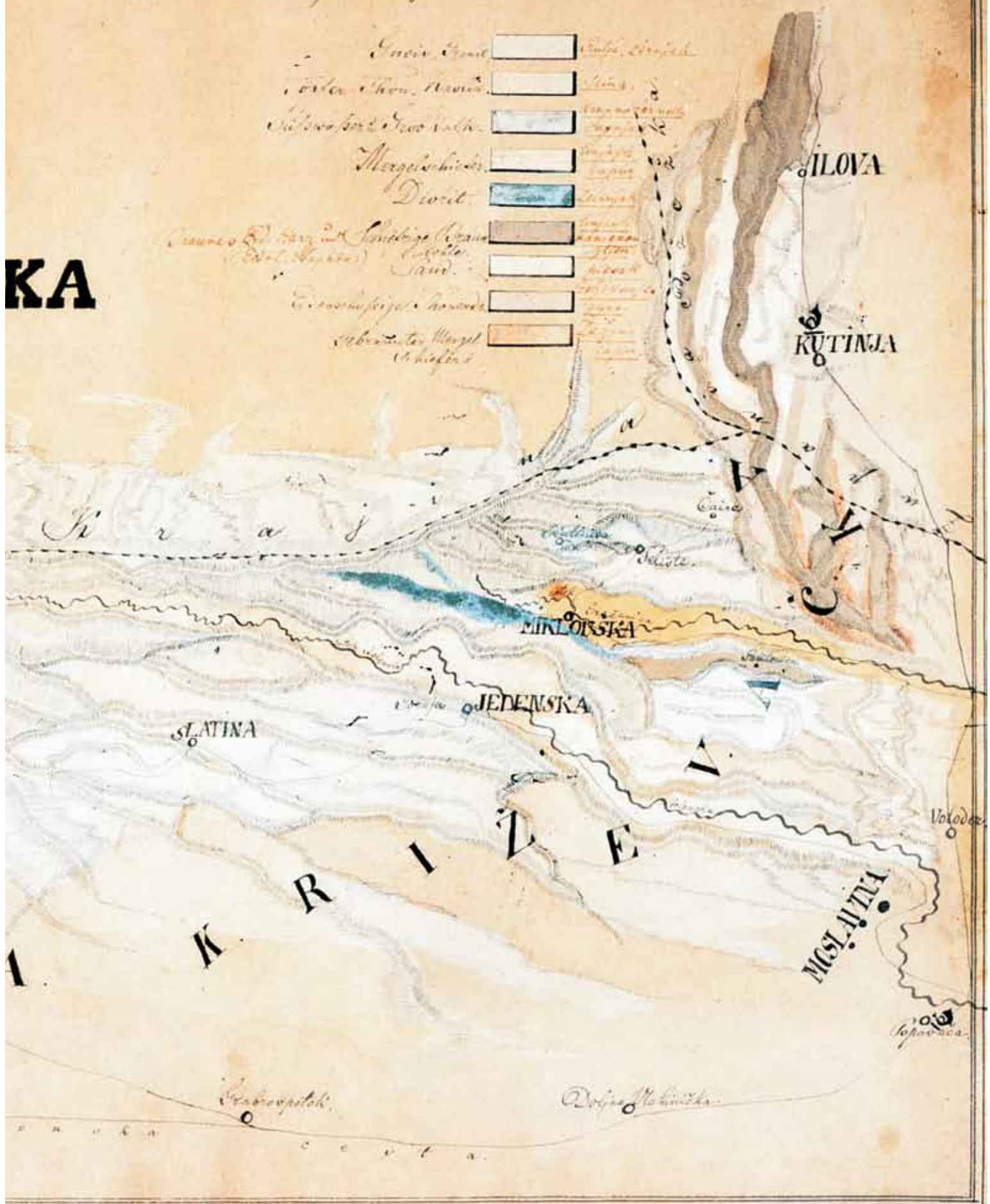
Sl. 1. Geološka karta Moslavačke gore (Vukotinić 1852)
