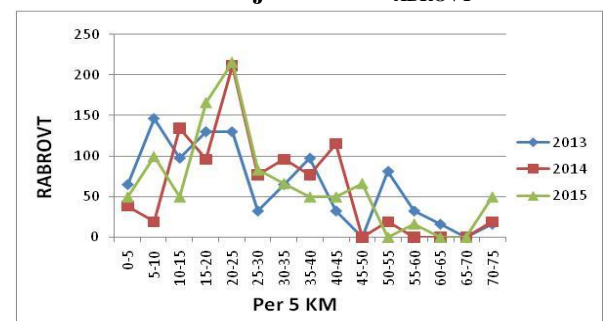
Gambar 15. Analisa angka kecelakaan berdasarkan kendaraan kilometer perjalanan (Accident Base Rate on Vehicle-km of Travel) pada jalan Trans Kalimantan Tahun 2013, 2014, dan 2015.
