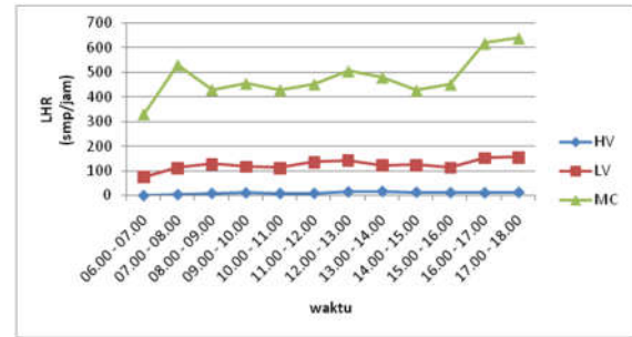
Gambar 9. Grafik LHR (smp) vs Waktu pada Segmen A Tahun 2015
