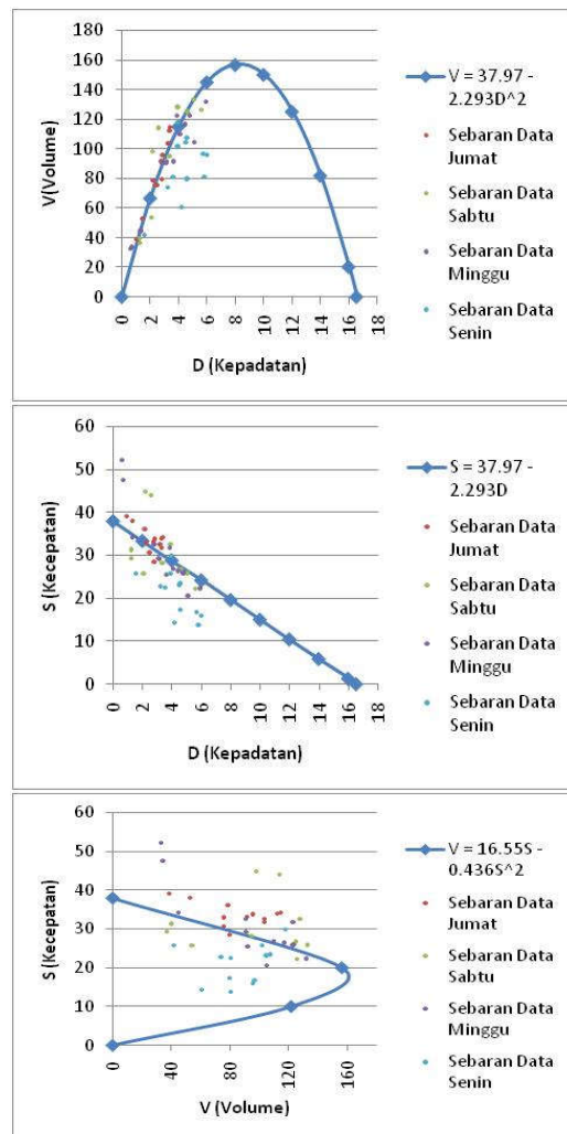
Gambar 10. Grafik Hubungan Volume, Kecepatan dan Kepadatan Kendaraan Ringan pada Jalan Ampera
