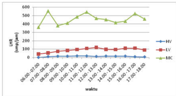
Gambar 8. Grafik LHR (smp) vs Waktu pada Segmen A Tahun 2015
