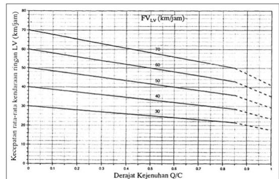
Gambar 1. Grafik Kecepatan sebagai fungsi dari Q/C untuk jalan 2/2 UD
