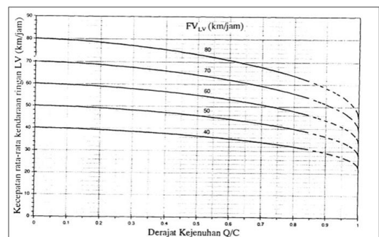
Gambar 2. Grafik Kecepatan sebagai fungsi dari Q/C untuk jalan empat lajur
