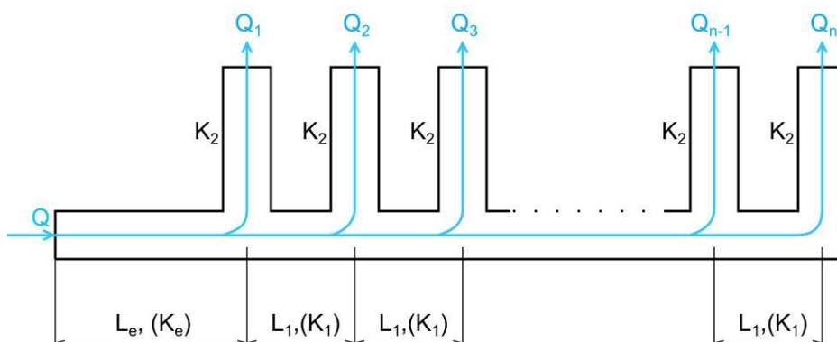
Obrázek I. Poddrážkový kanál který napájí řadu radiálních kanálů[2]
