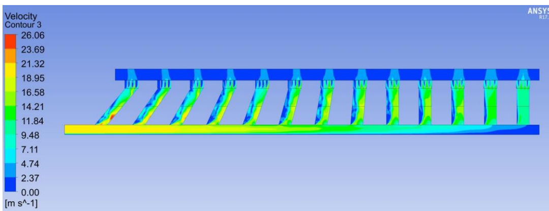
Obrázek V. Rozložení rychlosti – varianta A
