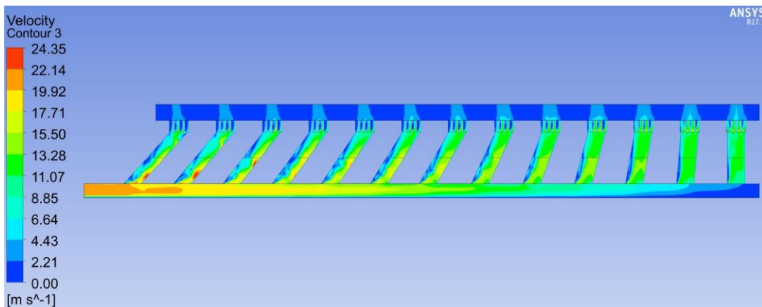
Obrázek V. Rozložení rychlosti – varianta A
