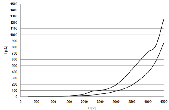
Obr. 9: V-A charakteristika - ECP VonRoll 217.22
