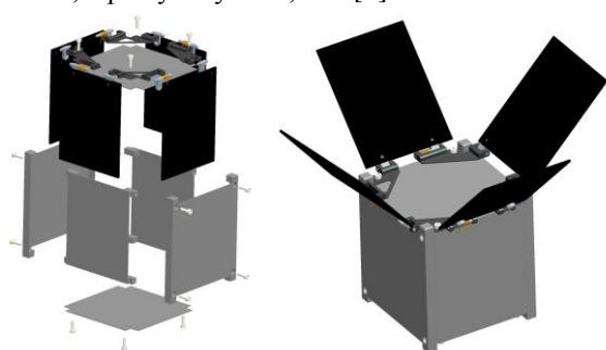
Obr. 1: Těleso pikosatelitu PilsenCUBE.
