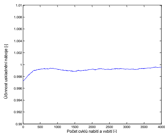
Obr. 3: Účinnost uskladnění náboje v superkapacitoru.
