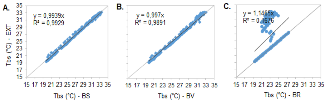
Figura 22. Relação funcional da temperatura de bulbo seco (Tbs; °C) entre ambiente externo e as baias sem climatização (BS; A), com ventilação forçada (BV; B) e resfriamento evaporativo (BR; C).
