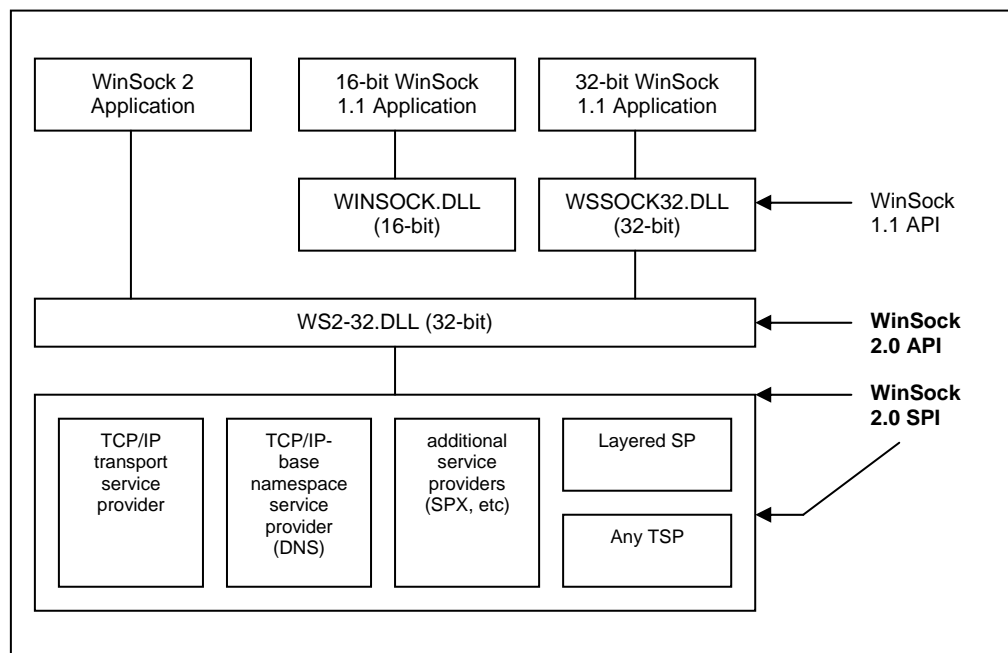
Gambar 3. Arsitektur WinSock 2
