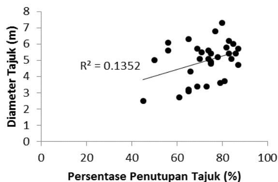
Gambar 2. Hubungan antara peubah persentase penutupan tajuk ( C ) dan rata-rata diameter tajuk ( \bar{D}_c )
