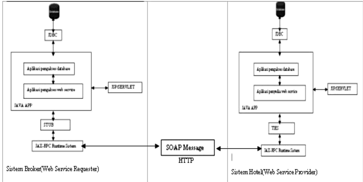
Gambar 3. Arsitektur Sistem
