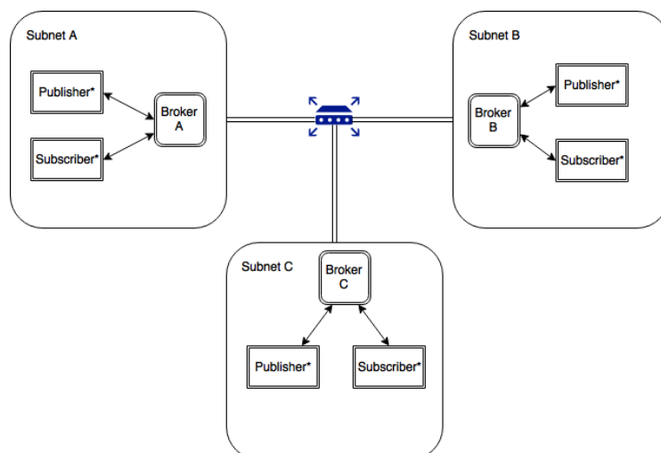
Gambar 10. Topologi Jaringan Pengujian
