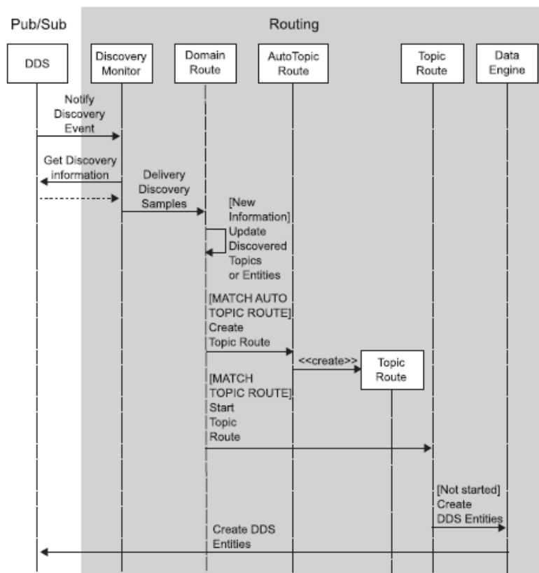
Gambar 6. Diagram Sekuens pada Proses Discovery Event
