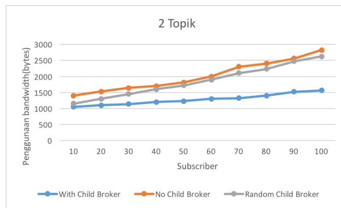
Gambar 15. Hasil Pengujian Penggunaan Bandwidth Broker untuk 2 Topik
