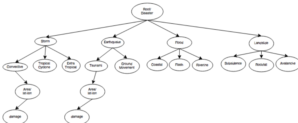
Gambar 9. Klasifikasi Hierarki
