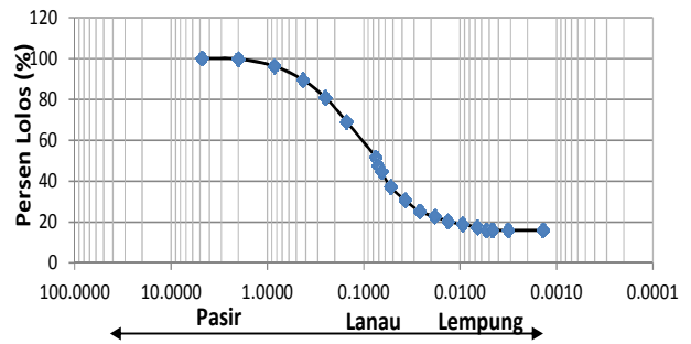
Gambar 4. Distribusi Ukuran Butiran Tanah Asli
