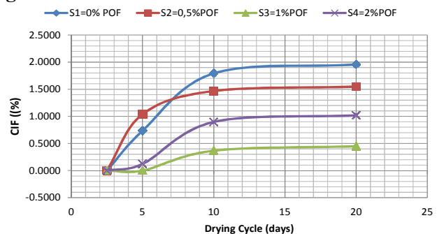
Gambar 9. Intensitas Keretakan Tanah (CIF) Pada Siklus Pengeringan
