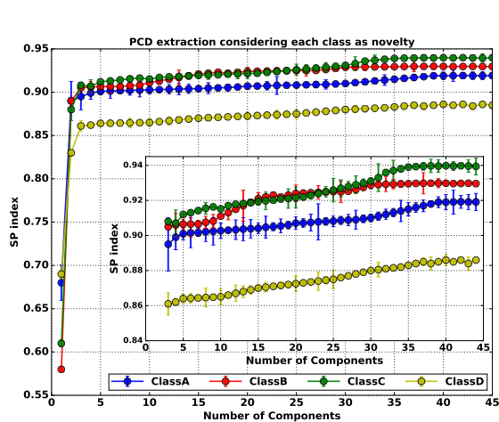
(a) Variação do Índice SP pela variação no número de componentes de discriminação extraídos por deflação. Cada linha colorida no gráfico representa o resultado para uma classe sendo tratada como novidade. A linha em azul representa o resultado obtido para a Classe A sendo tratada como classe novidade. Já a linha em vermelho representa o resultado para a Classe B como classe novidade. A linha em verde representa o resultado para a Classe C como novidade e, por fim, a linha amarela representa a o resultado obtido para a Classe D tratada como novidade. No detalhe, os pontos mais relevantes dos gráficos anteriores são apresentados.
