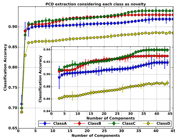
(b) Variação do Acurácia de Classificação pela variação do número de componentes de discriminação extraídos por deflação. Cada linha colorida no gráfico representa o resultado para uma classe sendo tratada como novidade. A linha em azul representa o resultado obtido para a Classe A sendo tratada como classe novidade. Já a linha em vermelho representa o resultado para a Classe B como classe novidade. A linha em verde representa o resultado para a Classe C como novidade e, por fim, a linha amarela representa a o resultado obtido para a Classe D tratada como novidade. No detalhe, os pontos mais relevantes dos gráficos anteriores são apresentados.
