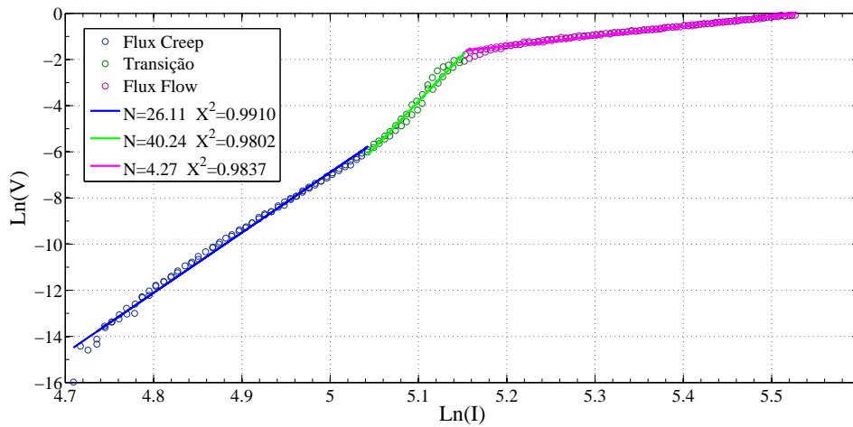
Figura 5.22: Curva Ln(V-I) da caracterização com pulsos de 100 ms por 2000 ms para fita Super Power modelo SCS4050-API.
