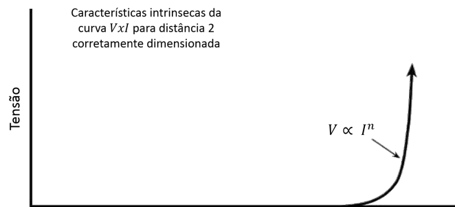
(a) Curva V-I típica de uma amostra supercondutora para um comprimento de transferência de corrente longo
