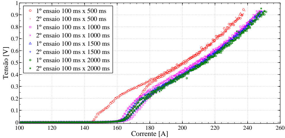
Figura 5.21: Curva V-I para fita da Super Power modelo SCS4050-API.
