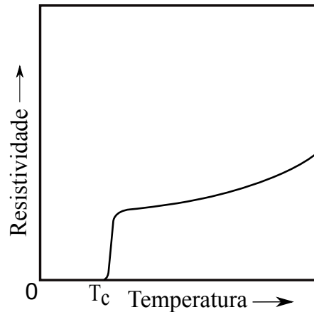
Figura 2.1: Perda da resistência para supercondutores a temperaturas criogênicas.
