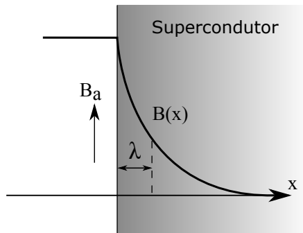
Figura 2.7: Variação da densidade de Fluxo nas Fronteiras de um Supercondutor.
