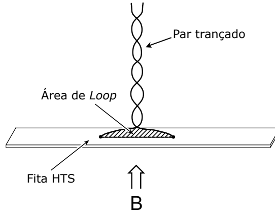
Figura 3.11: Par trançado dos fios de tensão e a área de loop no contato com a amostra
