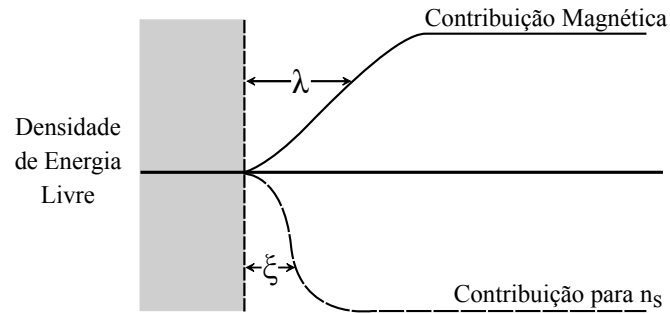
(a) Profundidade de penetração e comprimento de coerência na fronteira
