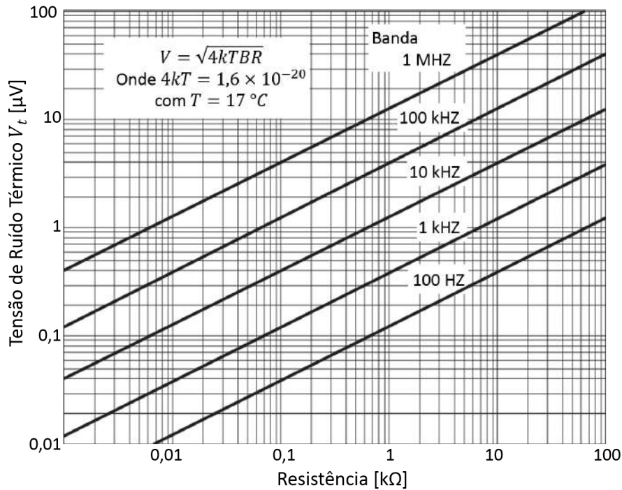
Figura 3.8: Ruído de Tensão térmica em função da resistência e banda de frequência. Figura adaptada de [57].
