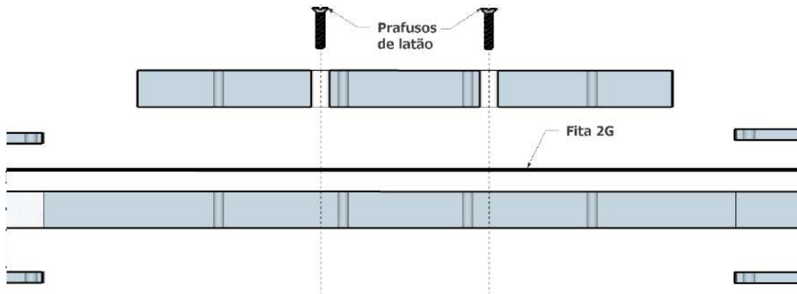
Figura 4.4: Vista ampliada do corte interno mostrando encaixe dos parafusos de latão na fita 2G para os contatos de tensão do método 4 pontas.
