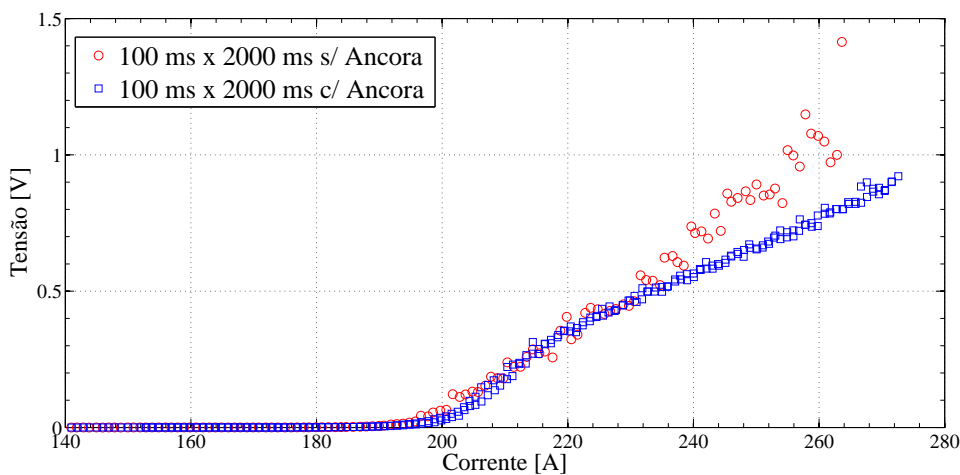
Figura 5.11: Curvas V-I para SuNam HCNK04150 sem camada de Kapton ® caracterizadas com pulsos 100 ms x 2000 ms com e sem ancoragem térmica.
