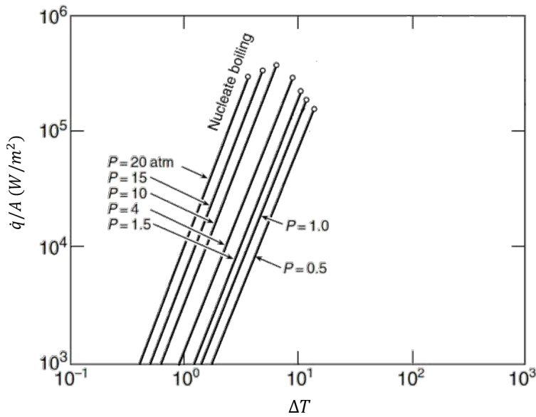
Figura 4.1: Curvas de nucleate-boiling para pressões diversas mostrando a transferência de calor de uma superfície metálica para nitrogênio líquido. O fluxo de calor crítico é previsto pelo círculo no topo das curvas de nucleate-boiling . Figura adaptada de [67].
