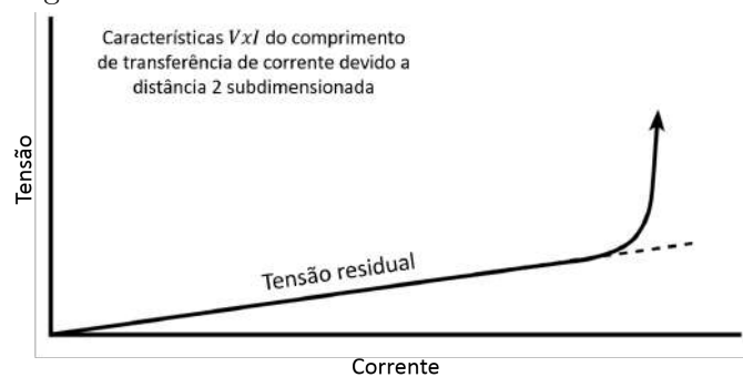
(b) Característica da curva V-I alterada linearmente por um comprimento de transferência de potência pequeno
