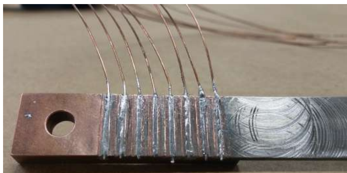
Figura 4.17: Fios de NbTi soldados no terminal de 4 K com solda de PbSn.
