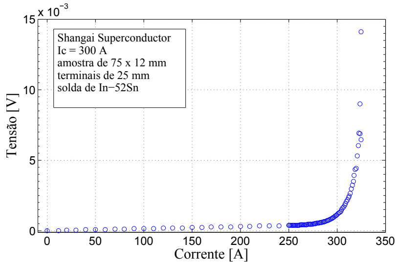
Figura 5.28: Curva V-I da amostra de 75 mm de comprimento da fita de 12 mm da Shanghai Superconductor lamina em inox 316 soldada em terminais de cobre.
