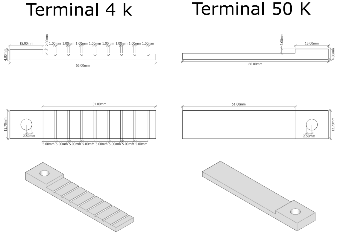
Figura 4.14: Projeto dos terminais de corrente dos current leads dimensionados para minimizar a resistência de contato e permitir extração de calor. Terminal de 4 K à esquerda com ranhuras para os fios de NbTi e terminal de 50 K à direita sem ranhuras.
