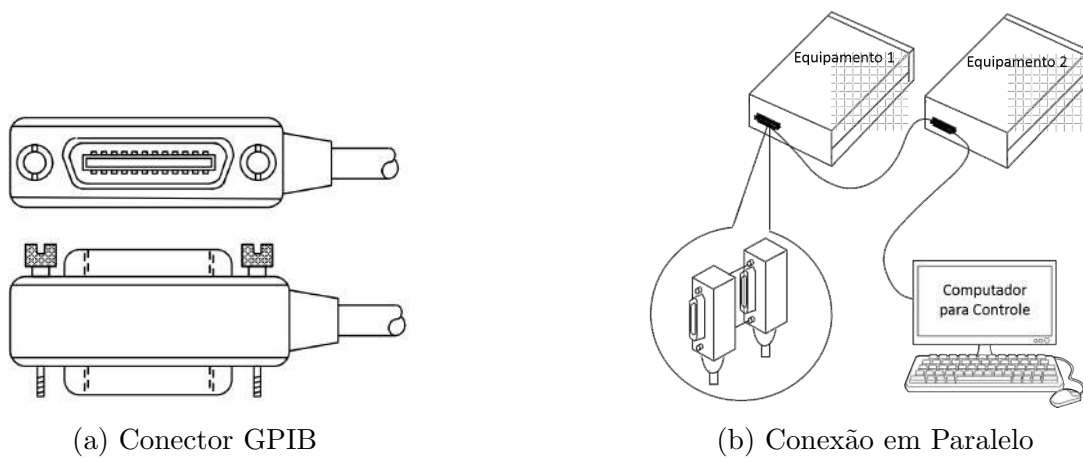
Figura 4.7: Barramento IEEE-488 para múltiplos equipamentos controlados por um computador.
