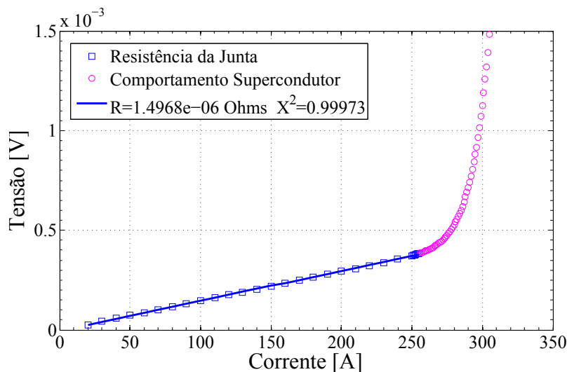
Figura 5.29: Curvas V-I para resistência de contato na amostra de 75 mm de comprimento da fita de 12 mm da Shanghai Superconductor lamina em inox 316
