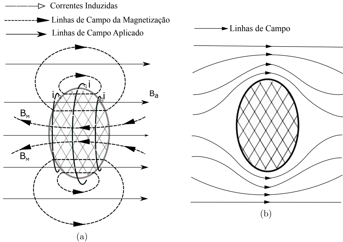
Figura 2.3: Distribuição do fluxo magnético em um condutor perfeito. (a) Sobreposição da densidade de campo aplicada B_a com a densidade de campo B_M gerada pelas correntes i de blindagem. (b) Corpo blindado do campo externo. Figura adaptada de [8].
