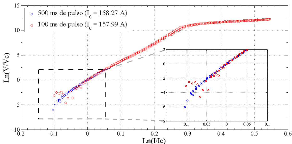
Figura 5.16: Curvas \text{Ln}(V-I) SuNam modelo HCNK04150 sem camada de Kapton ® para ensaios de 100 ms e 500 ms de pulso sobrepostas.
