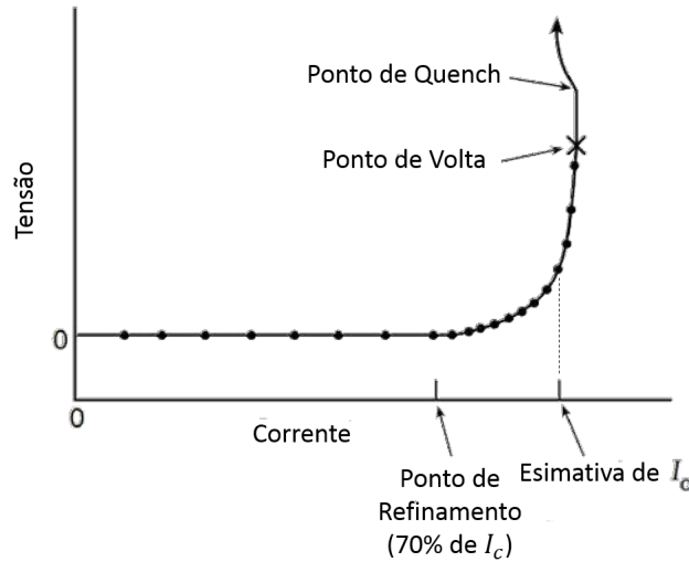
Figura 3.14: Esboço de um gráfico tensão x corrente típico de um supercondutor, mostrando região resistência negligenciável ( < 70\% I_c ), a região altamente não linear próxima da corrente crítica e o ponto de quench .
