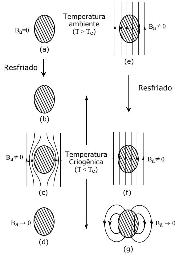
Figura 2.4: Comportamento Magnético de um Condutor Perfeito. (a)-(b) Condutor perde a resistência na ausência de campo. (c) Densidade de campo é aplicada ao condutor sem resistência. (d) Campo é removido. (e)-(f) Condutor perde a resistência na presença de campo. (g) Densidade de campo externa aplicada é removida. Figura adaptada de [8].
