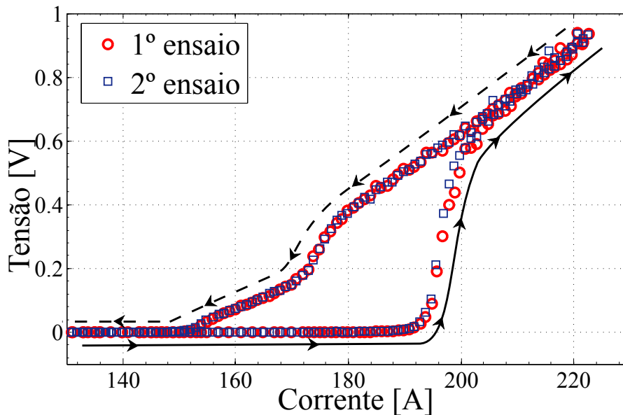
Figura 5.3: Curva V-I para fita da SuNam modelo HCNK04150 com camada de Kapton ® caracterizada com 100 ms x 500 ms e E_{stop} = 2e5 \times E_c .
