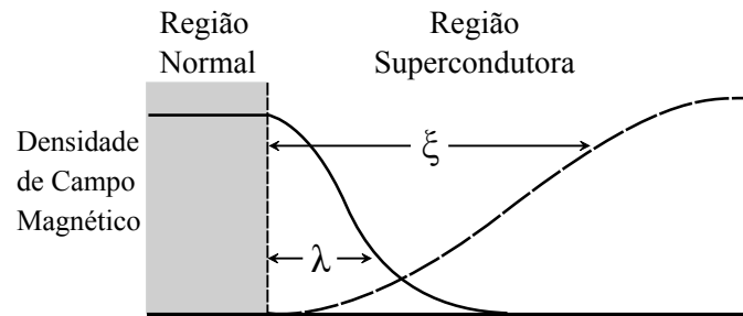
(a) Profundidade de penetração e comprimento de coerência na fronteira
