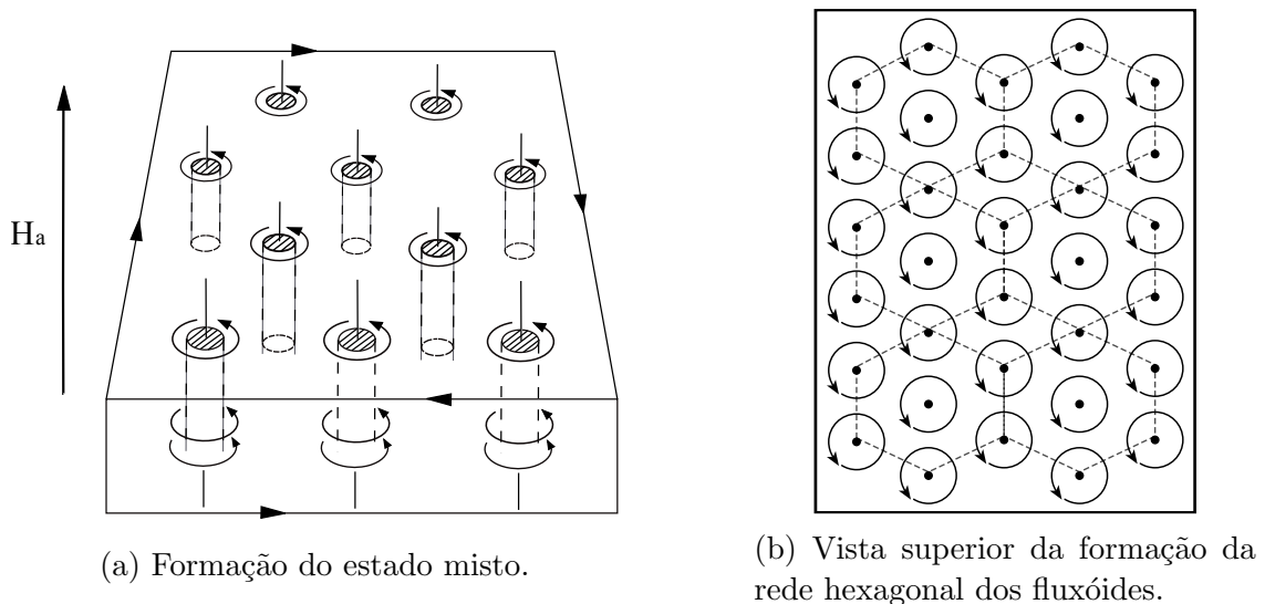
Figura 2.10: Formação dos fluxóides e vórtices de corrente no estado misto. Figura adaptada de [2].
