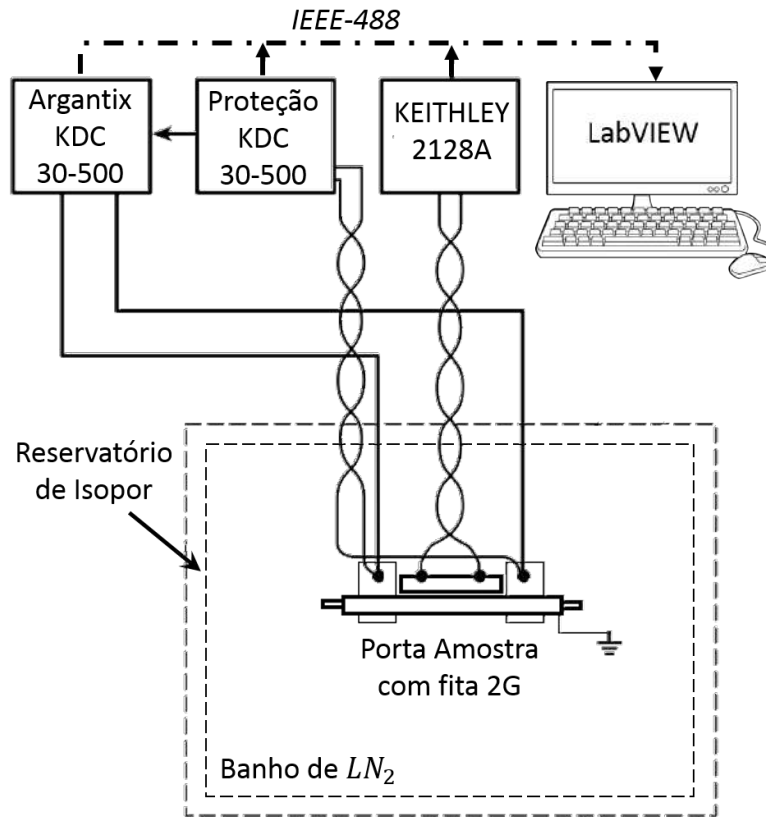
Figura 4.8: Diagrama da conexão dos equipamentos utilizados no sistema de caracterização.
