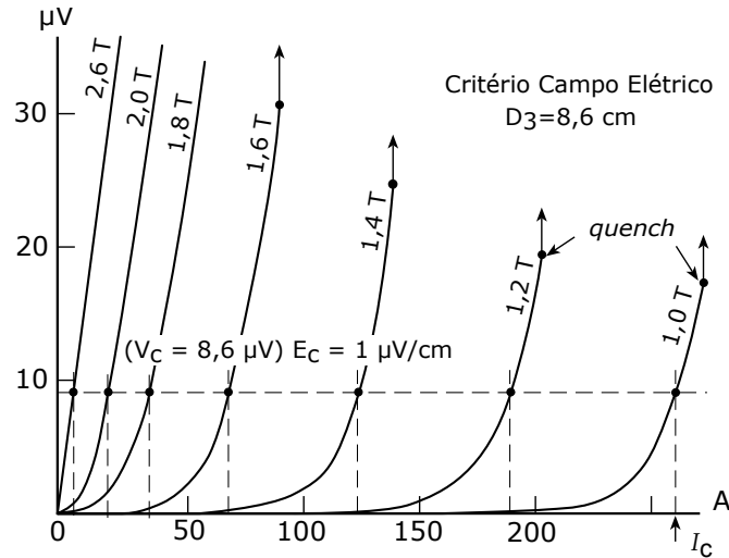
Figura 3.18: Curvas V - I hipotéticas para diferentes campos magnéticos utilizando o critério do campo crítico. Figura adaptada de [53].
