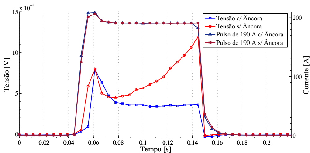
Figura 5.24: Curvas de tensão e corrente para pulsos de 100 ms e 190 A as situações de porta amostra com e sem ancoragem térmica.
