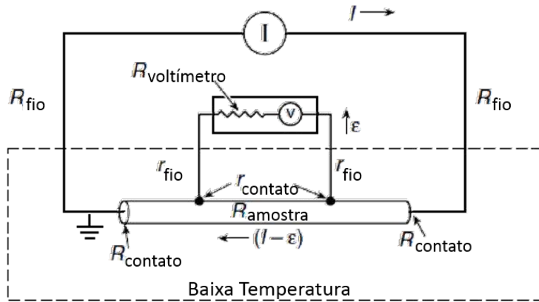
(b) Arranjo quatro pontas para medição de corrente de transporte.
