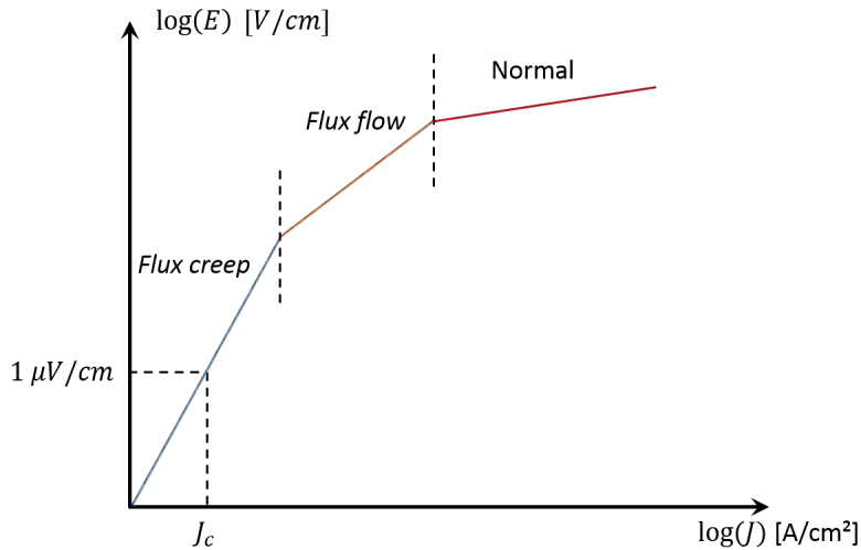
Figura 2.17: Influência do fator exponencial N na relação E-J
