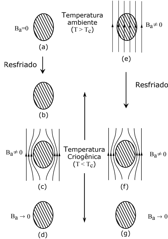
Figura 2.5: Comportamento Magnético do Supercondutor. (a)-(b) Condutor perde a resistência na ausência de campo. (c) Densidade de campo é aplicada ao condutor sem resistência. (d) Campo é removido. (e)-(f) Condutor perde a resistência na presença de campo. (g) Densidade de campo é removida. Figura adaptada de [8].
