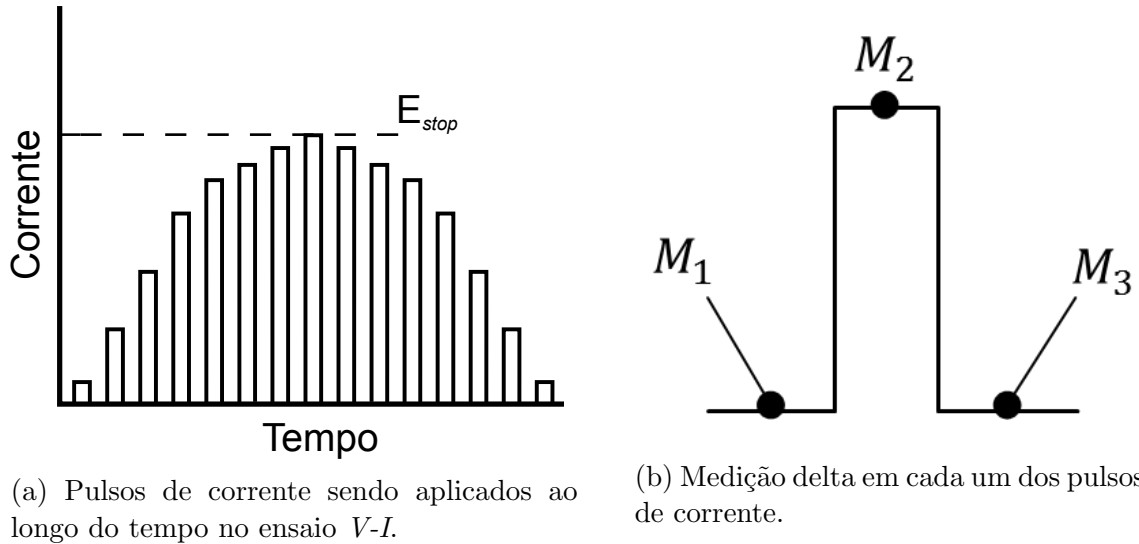
Figura 3.17: Ensaio de caracterização V - I usando corrente pulsada.
