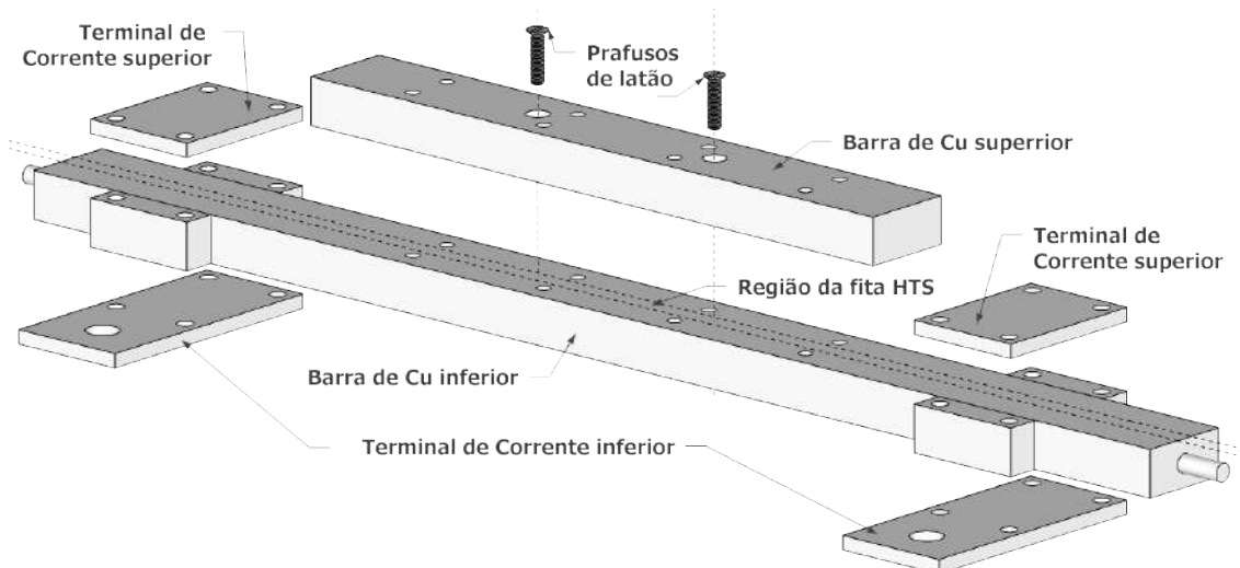
Figura 4.2: Design para o porta amostra com ancoragem térmica.
