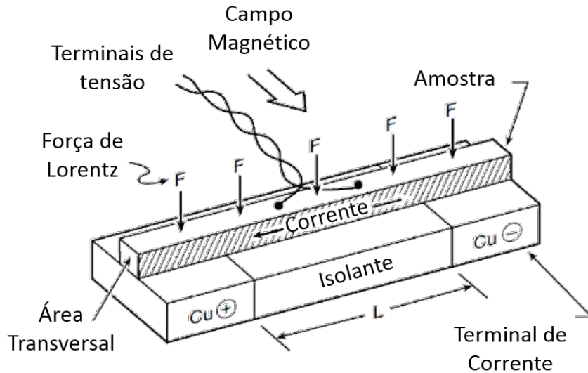
Figura 3.1: Imagem adaptada de [53]. Exemplo de um porta amostra simples para medição de pequenas amostra de supercondutores de alta corrente.
