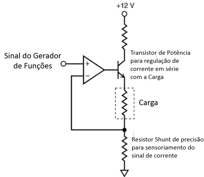
Figura 3.16: Diagrama de um circuito linear básico de uma fonte de corrente regulada por transistor de potência. Figura adaptada de [53].
