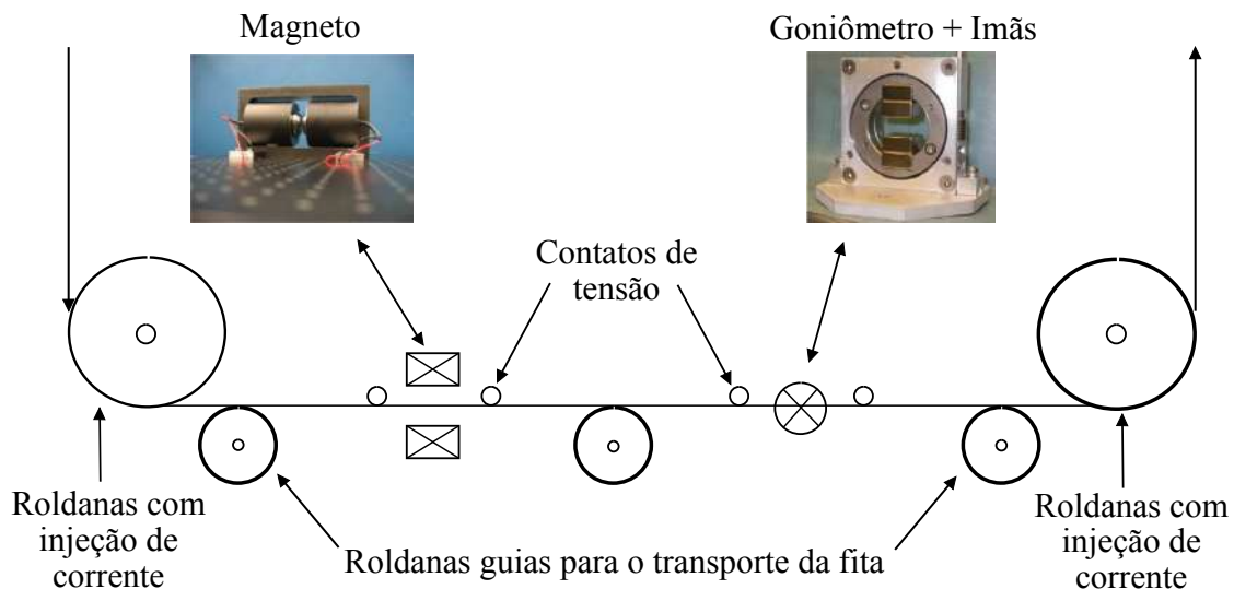
Figura 2.18: Esquemático do sistema de medição do Laboratório Nacional de Los Alamos. Figura adaptada de [34].
