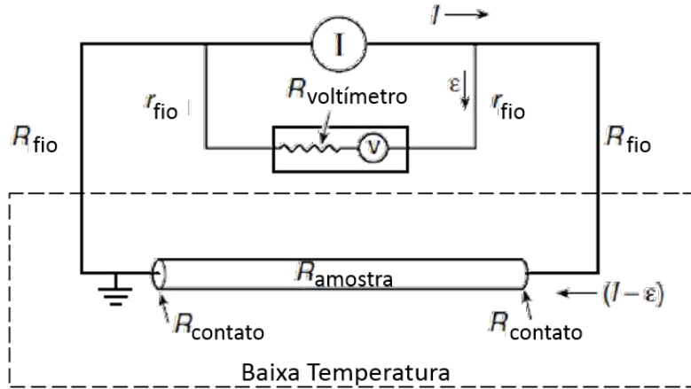
(a) Arranjo de duas pontas para medição de corrente de transporte.
