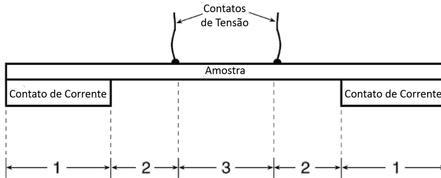
Figura 3.3: Distâncias relevantes nos contatos de corrente e tensão para medição da amostra
