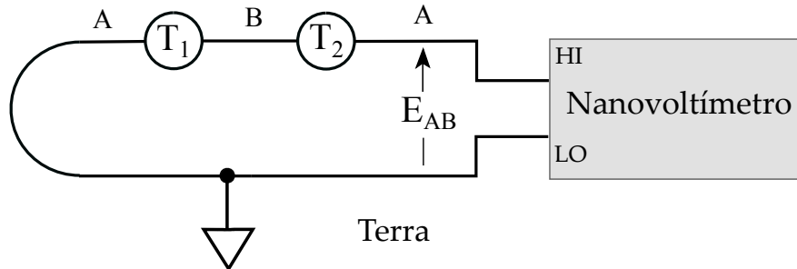
Figura 3.6: tensão termoelétrica gerada entre materiais A e B diferentes em série no circuito de medição. Figura adaptada de [56].
