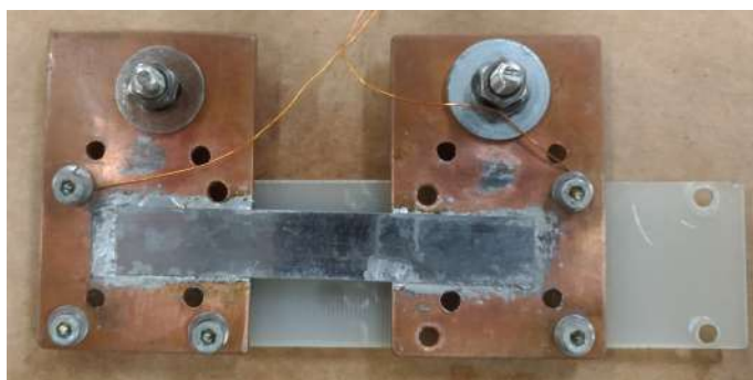
Figura 4.18: Suporte feito de G10 e duas chapas de cobre para teste de solda na fita de 12 mm da Shanghai Superconductor.
