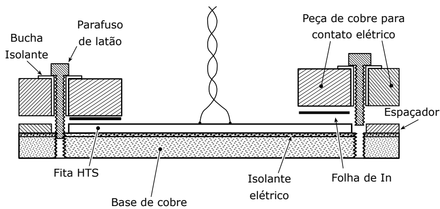
Figura 3.5: Contatos de pressão feitos em fita HTS com folha de In. O contato de corrente é feito com blocos de cobre livres de óxido, parafusados em uma base de cobre isolada para fazer pressão contra uma camada intermediária de folha de In e a superfície da fita. Figura adaptada de [53].
