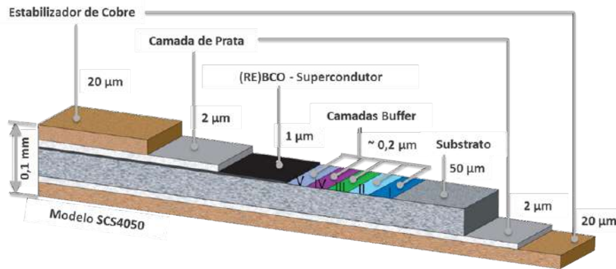
Figura 2.16: Corte laminar da fita Super Power 2G HTS SCS4050. Figura adaptada de [24].
