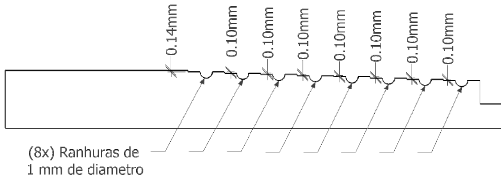
Figura 4.10: Detalhes das ranhuras no primeiro design do terminal de 4 K para encaixe dos fios de NbTi.
