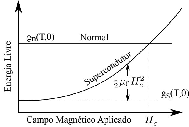
Figura 2.6: Efeito do campo magnético na energia livre de Gibbs
