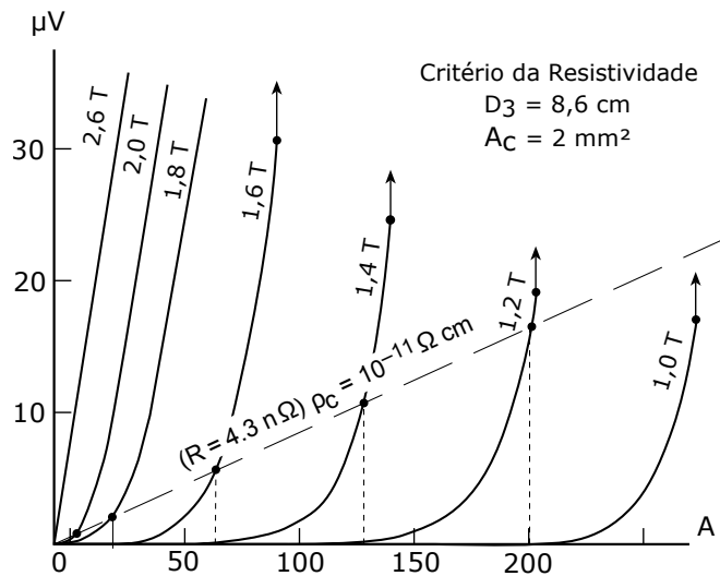
Figura 3.19: Curvas V - I hipotéticas para diferentes campos magnéticos utilizando o critério da resistividade. Figura adaptada de [53].
