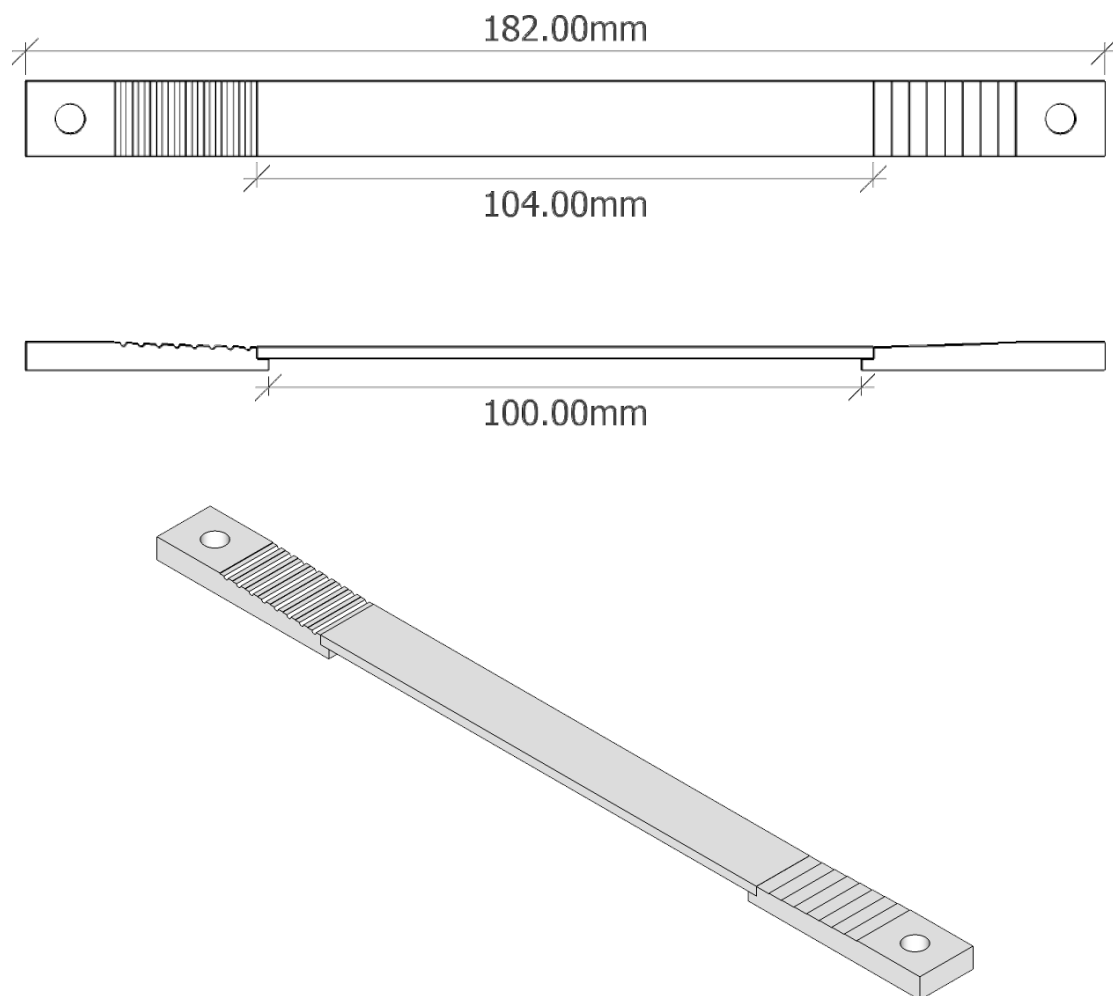
Figura 4.11: Montagem dos dois terminais 4K e 50 K com a barra de inox.
