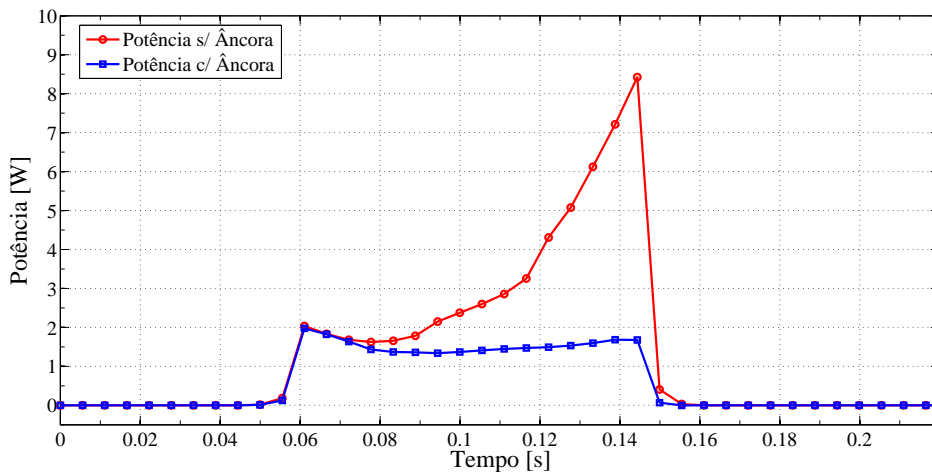
Figura 5.27: Curvas de potência dissipada em pulsos de 100 ms e 200 A nas situações de porta amostra com e sem ancoragem térmica.
