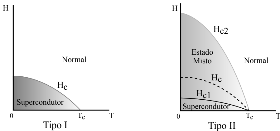
Figura 2.12: Diferença no comportamento magnético dos supercondutores do tipo I e do tipo II. Figura adaptada de [2].
