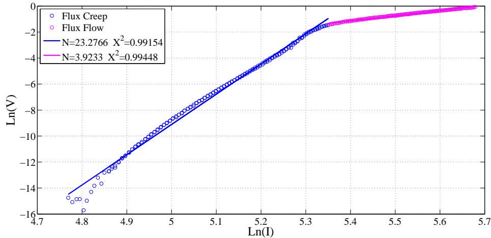
Figura 5.20: Curva Ln(V-I) da caracterização com pulsos de 100 ms por 2000 ms para fita SuperOx modelo 2014-10-R.
