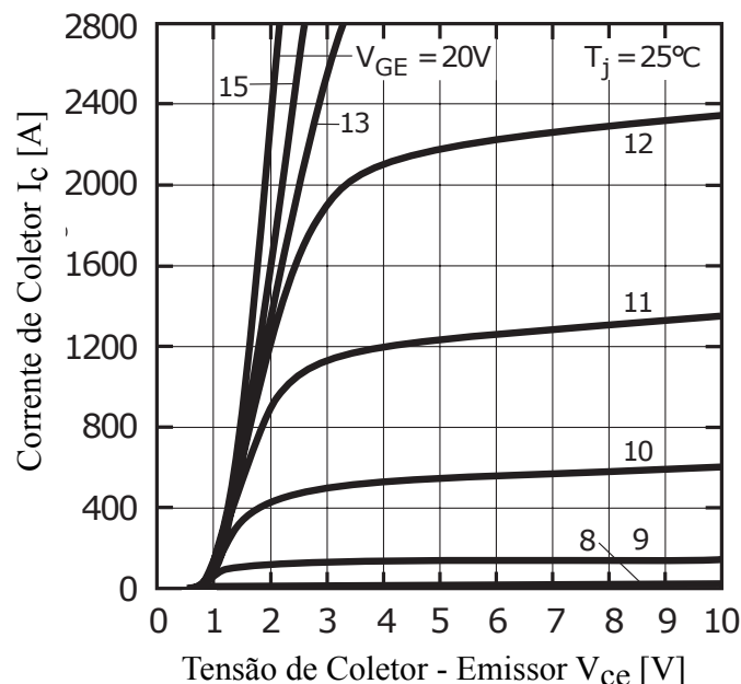
Figura A.2: Curvas típicas de operação do módulo IGBT CM1400DU-24NF da POWEREX. Figura adaptada do datasheet do fabricante.
