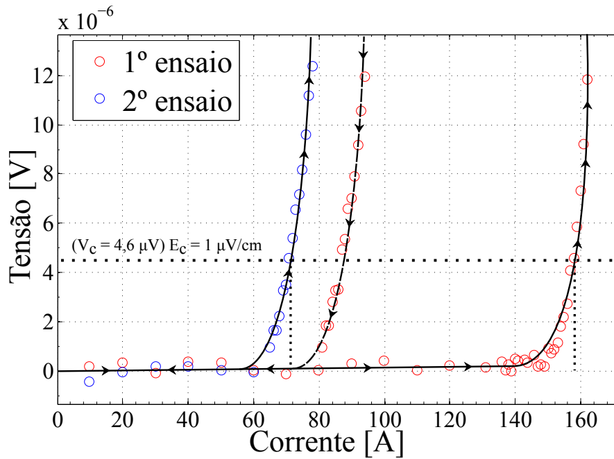
Figura 5.4: Análise V-I ampliando a Figura 5.3 próximo do valor de V_c .
