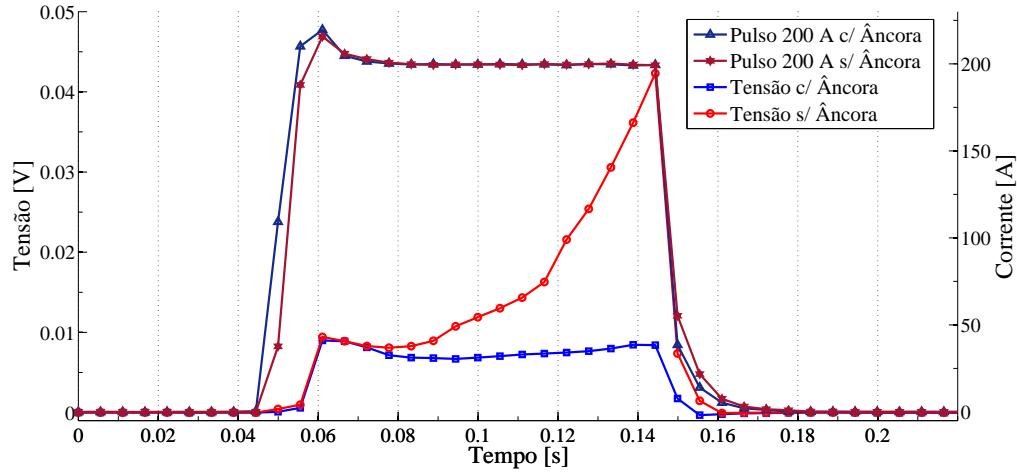
Figura 5.26: Curvas de tensão e corrente para pulsos de 100 ms e 200 A nas situações de porta amostra com e sem ancoragem térmica.
