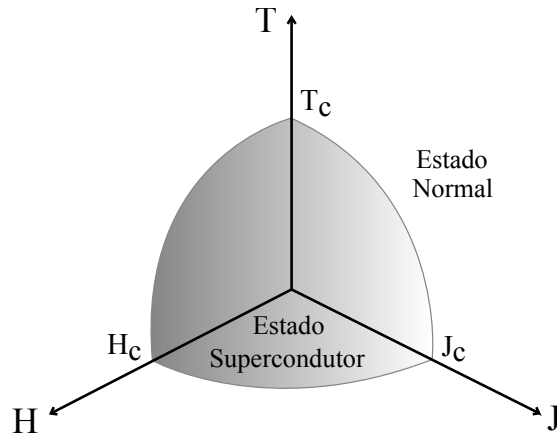
Figura 2.2: Estado supercondutor delimitado por seus parâmetros críticos T_c , H_c e J_c . Figura adaptada de [2].
