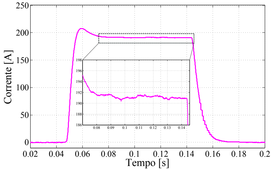
Figura 4.5: Pulso de corrente programado para 190 A e 100 ms de duração na fonte Argantix KDC 30-500.
