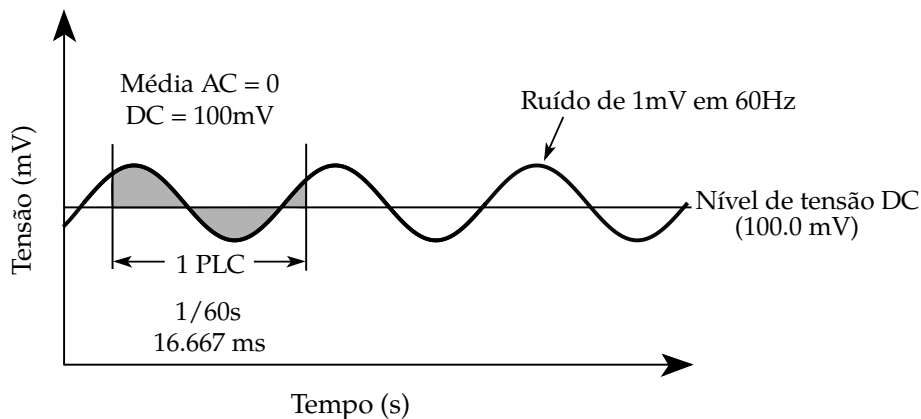
Figura 3.10: Integração em um ciclo de rede para retirar valor médio do ruído de 60 Hz. Figura adaptada de [56].
