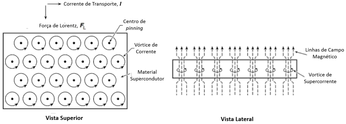
Figura 2.13: Supercondutor do tipo-II transportando corrente no estado misto.
