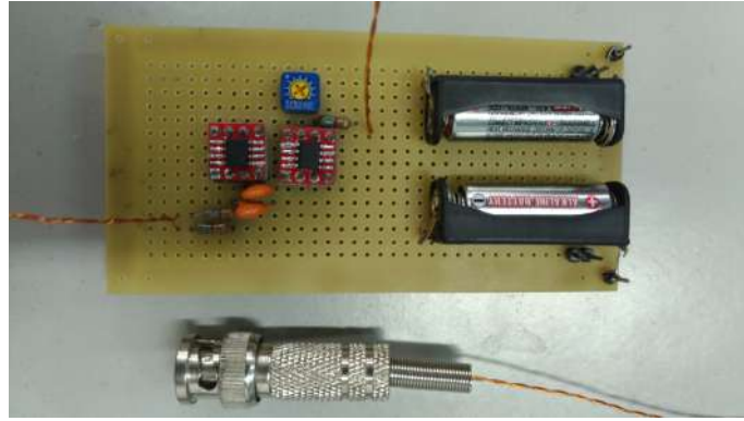
Figura A.4: Placa de pré-amplificação montada.
