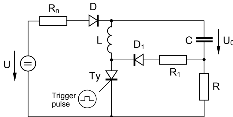
Figura 2.19: Esquemático adaptado de Frolek et al. [44] U é a tensão da fonte de alimentação; U_0 é a tensão no banco de capacitores; T_y é um tiristor. R_1 e R_n são resistores; D e D_1 são diodos; L é um indutor; C a capacitância do banco de capacitores; e R a amostra de material fita HTS.
