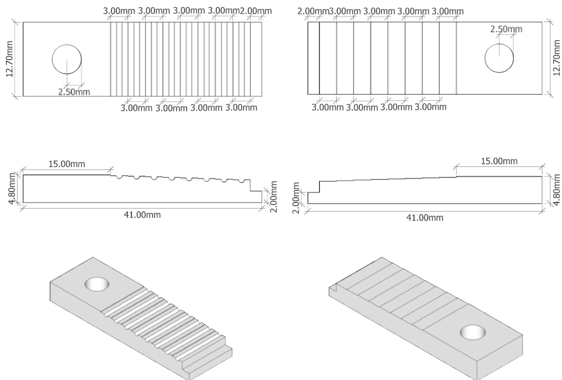
Figura 4.9: Projeto dos terminais de corrente do current lead para restrição espacial do criostato. Terminal de 4 K à esquerda com ranhuras para os fios de NbTi e terminal de 50 K a direita sem ranhuras.
