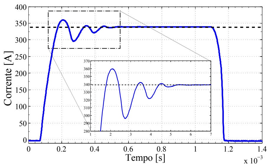
Figura 5.23: Pulso de de 1 ms e 340 A do circuito IGBT conectado ao porta amostra.
