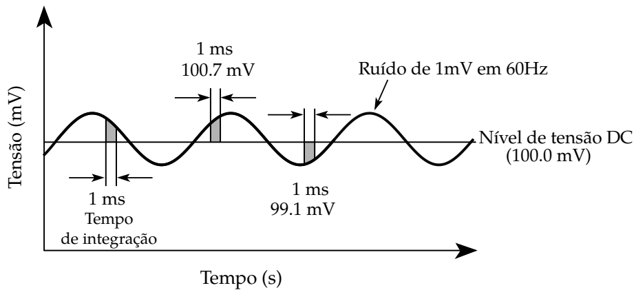
Figura 3.9: Ruído de rede de 1 mV superposto em um sinal de 100 mV CC. Figura adaptada de [56].
