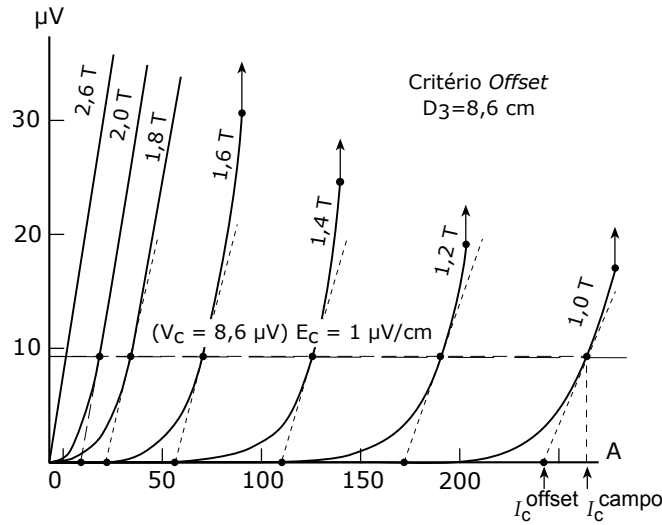
Figura 3.20: Curvas V-I hipotéticas para diferentes campos magnéticos utilizando o critério do Offset . Figura adaptada de [53].
