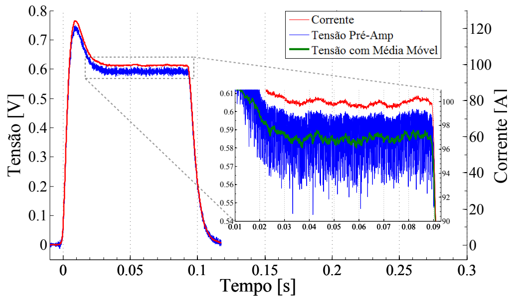
Figura A.5: Tensão de Resistor shunt monitorada pelo pré-amplificador com ganho 100 em um pulso de 100 A de 100 ms da fonte KDC 30-500.
