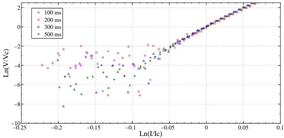
Figura 5.15: Curva logarítmica de V-I da região intrínseca para fita da SuNam modelo HCNK04150 sem camada de Kapton ® .
