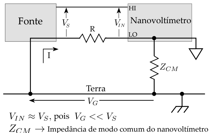
Figura 3.13: Redução de loops de terra com impedância de modo comum.
