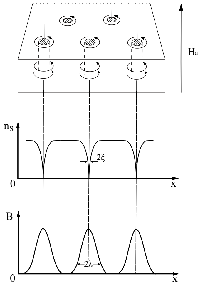
Figura 2.11: Dimensionamento dos fluxóides pelos parâmetros \lambda e \xi . Figura adaptada de [2].
