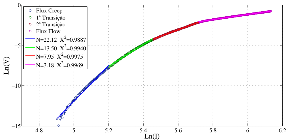
Figura 5.18: Curva Ln(V-I) da caracterização com pulsos de 100 ms por 2000 ms para fita Shanghai Superconductors.
