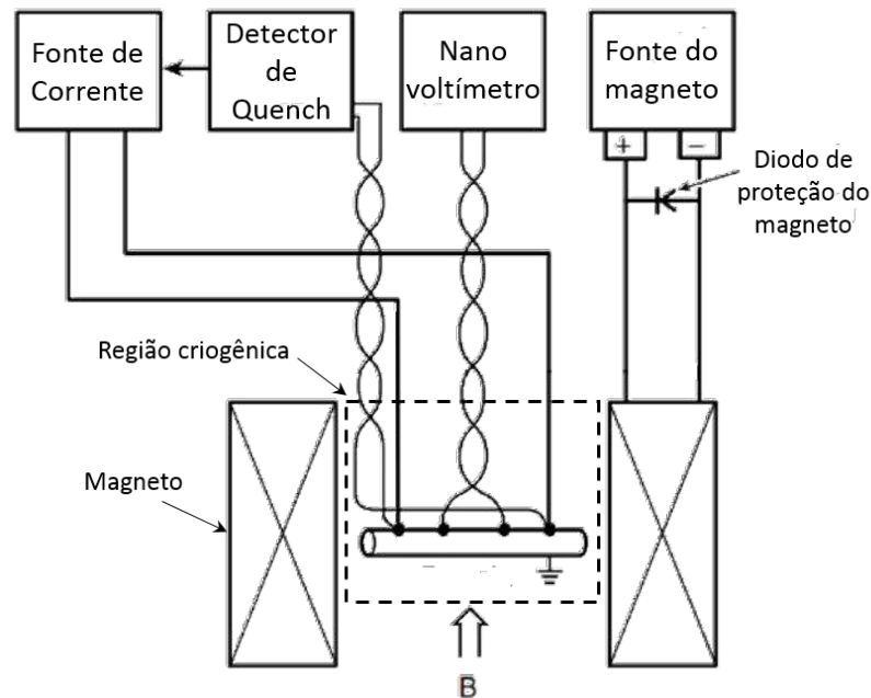
Figura 3.15: Diagrama da instrumentação para medição de corrente crítica.
