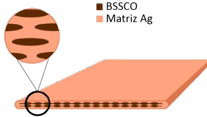
Figura 2.15: Estrutura multifilamentar da fita 1G. Figura adaptada do site da fabricante SuperOx ( http://www.superox.ru/en/ ).
