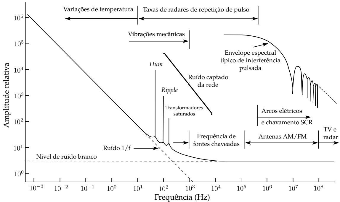
Figura 3.7: Espectro de frequência das fontes de ruído de tensão. Figura adaptada de [57].
