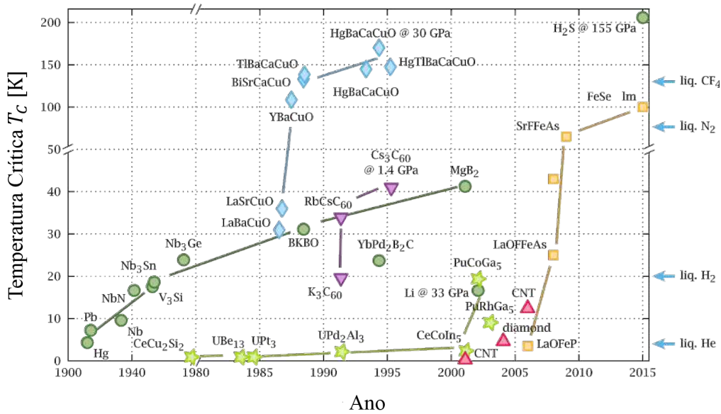
Figura 2.14: Linha cronológica da descoberta de materiais supercondutores até os dias atuais. Figura retirada de [20].
