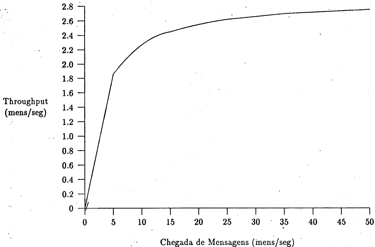
Figura 4: Throughput do Bit Alternante
