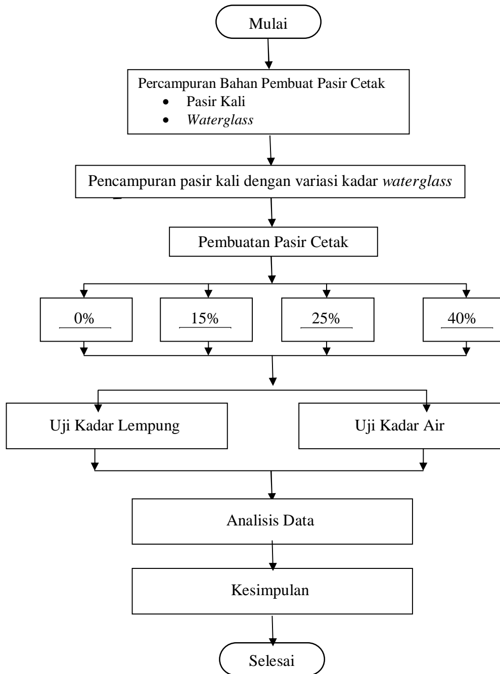
Gambar 1. Bagan Alir Proses Eksperimen
