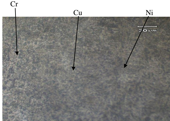
Gambar 8. Foto Struktur Mikro Daerah Lasan Pengelasan MIG Plat 316 Etsa Kalling ReagentPembesaran 400x
