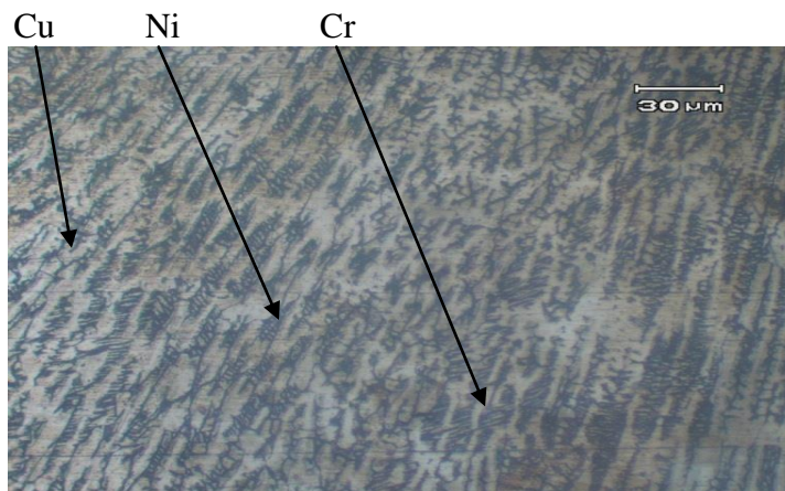
Gambar 7 Foto Struktur Mikro Daerah Lasan Pengelasan TIG Plat 304 Etsa Kalling Reagent Pembesaran 400x
