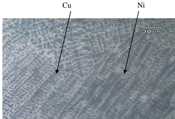
Gambar 6. Foto Struktur Mikro Daerah Lasan Pengelasan TIG Plat 316 Etsa Kalling Reagent Pembesaran 400x
