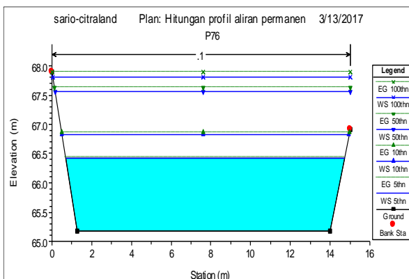
Gambar 10. Profil Melintang di titik P76
