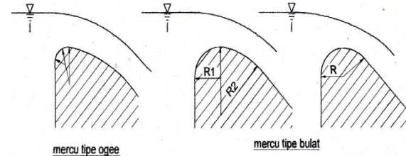
Gambar 1. Bentuk mercu bendung
