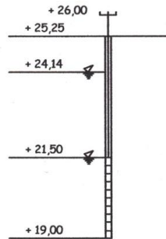
Gambar 6. Ukuran pintu pembilas
