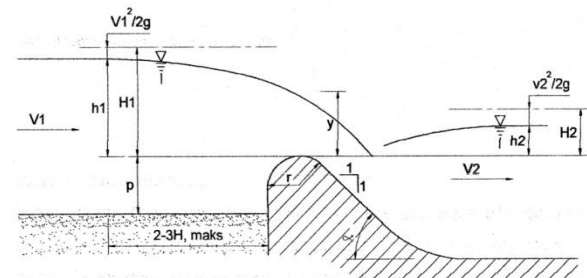
Gambar 2. Bendung dengan mercu bulat
