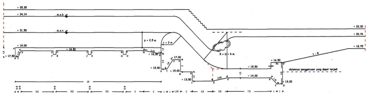
Gambar 5. Konstruksi Bendung
