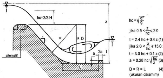
Gambar 3. Kolam Olakan menurut Vlugter
