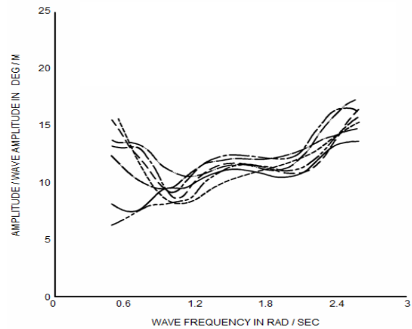
Figure 5. Response of Pitch Motion. Monohull (—), Catamaran S/L 0.2 (---), Catamaran S/L 0.3 (---), Catamaran S/L 0.4 (---), Trimaran S/L 0.2 (----), Trimaran S/L 0.3 (---), Trimaran S/L 0.4 (----)
