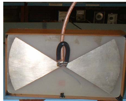
Gambar 4. Foto antena Bowtie ujung Sirkuler yang diimplementasikan
