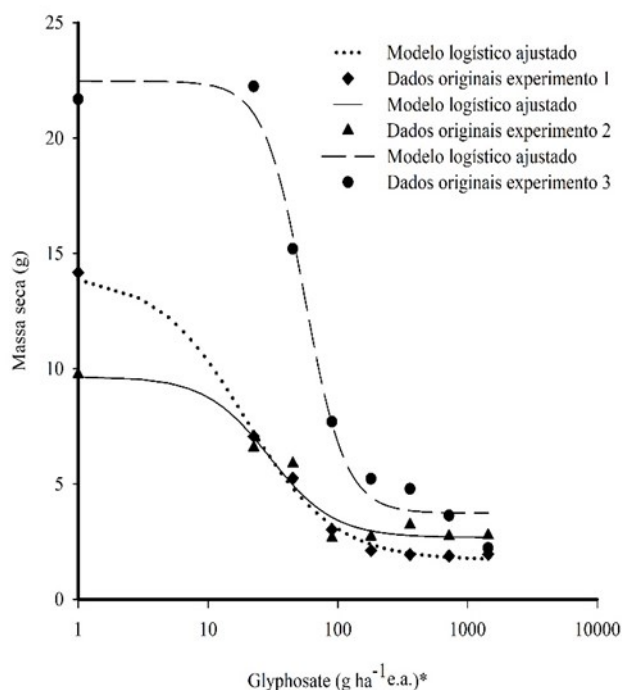
Figura 1. Modelos de regressão não-linear logísticos ajustados para massa seca (g) de plantas de U. decumbens aos 21 DAA em função das doses de glyphosate (g ha -1 e.a.).
