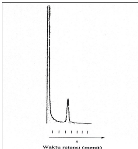
Gambar 3. Kromatogram d-aletrin dengan waktu retensi 3,28 menit
