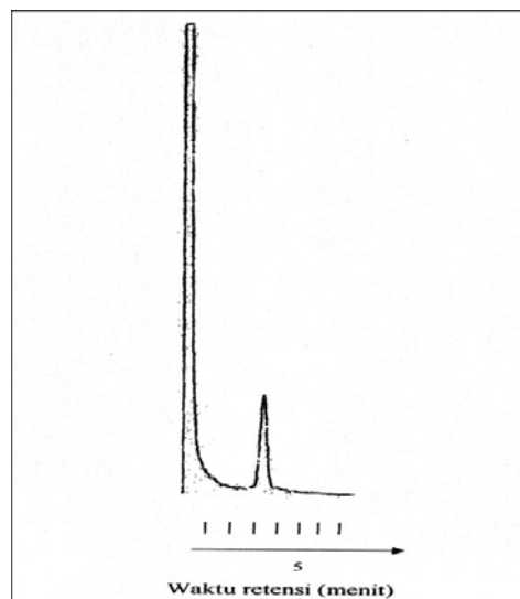
Gambar 4. Kromatogram sampel d-aletrin dengan waktu retensi 3,28 menit
