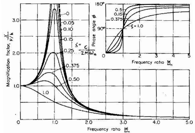
Gambar 5. Respon getaran untuk satu derajat kebebasan [8].
