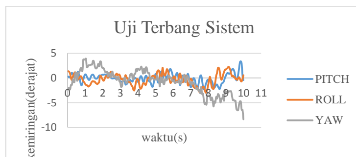
Gambar 9 Grafik hasil uji terbang
