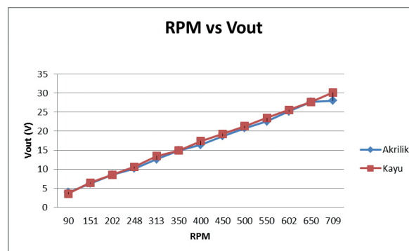
Gambar 10. Grafik perbandingan tegangan keluaran cakram kayu dan akrilik.
