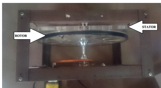
Gambar 7. Kerangka Generator Axial Tampak Atas Sumber: Dokumentasi pribadi
