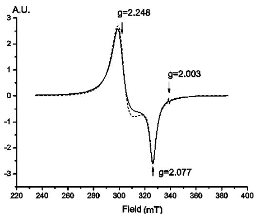
Рис. 6. Спектр ЭПР (сплошная линия) образца Cu-СЭЛ после химической трансформации в процессе хранения (содержание меди 7.9 % масс.; T_{\text{изм}} 25 °С) и модельный спектр ЭПР (пунктирная линия)
