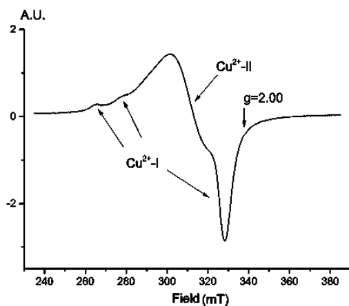
Рис. 3. Спектр ЭПР образца Cu-СЭЛ (содержание меди 3.8 % масс.; T_{\text{изм}} 25 °C)
