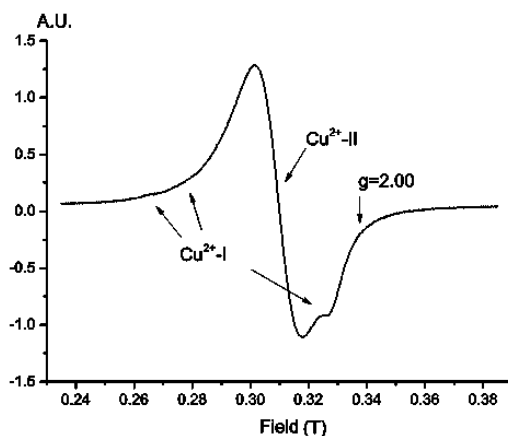
Рис. 5. Спектр ЭПР образца Cu-СЭЛ (содержание меди 7.9 % масс.; T_{\text{изм}} 25 °С)
