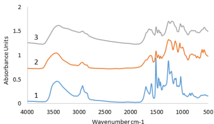
Рис. 1. ИК-спектры образцов: 1 – этанолигнин пихты; 2 – аммонийная соль сульфатированного этанолигнина пихты; 3 – медьсодержащий сульфатированный этанолигнин пихты
