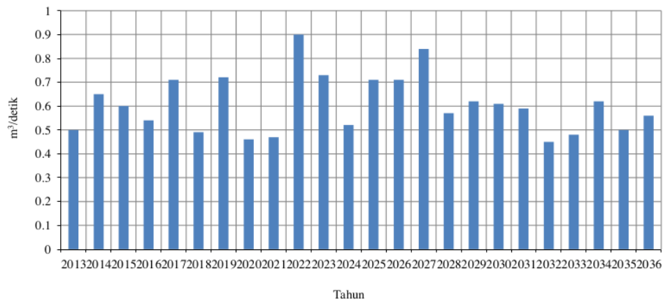
Gambar 3. Debit rata-rata bangkitan (m 3 /det)
