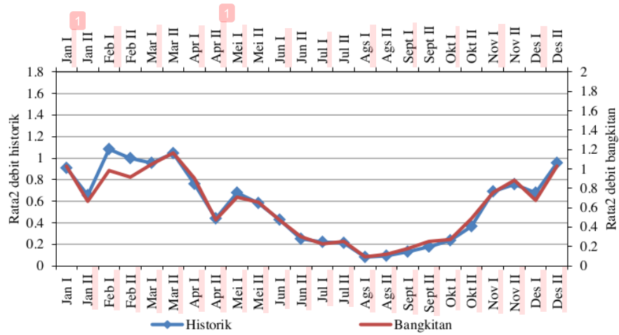
Gambar 5. Parameter statistik rata-rata antara debit historik dengan debit bangkitan
