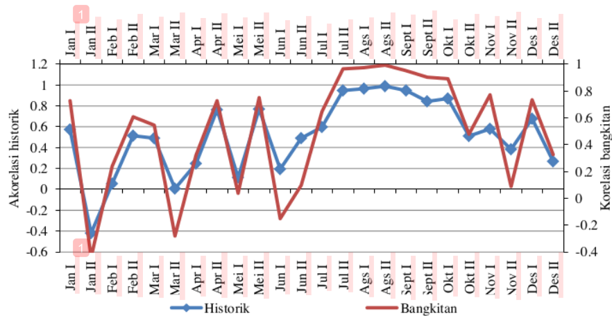
Gambar 7. Parameter statistik korelasi antara debit historik dengan debit bangkitan
