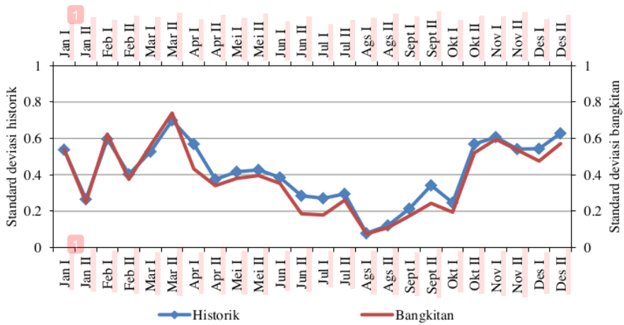
Gambar 6. Parameter statistik standar deviasi antara debit historik dengan debit bangkitan
