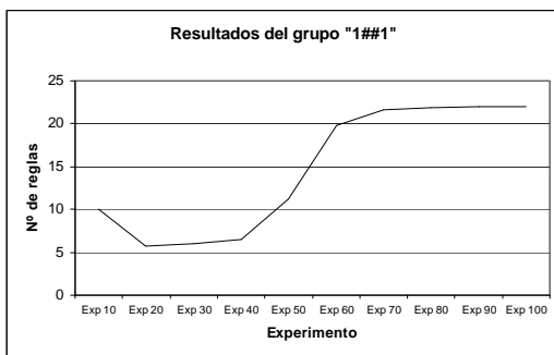
Figura 15: Evolución del número de reglas del grupo "1##1" con el aumento de aleatoriedad en la generación del tablero.
