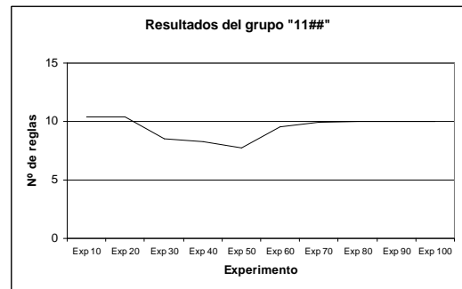
Figura 14: Evolución del número de reglas del grupo "11##" con el aumento de aleatoriedad en la generación del tablero.
