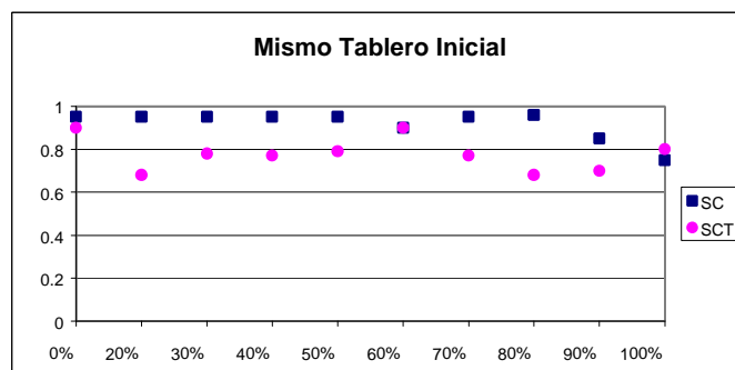
Figura 6: Tanto por ciento de partidas ganadas por el SCT y el SC clásico, promediando sobre 5 situaciones distintas, desde el mismo tablero inicial, frente a un jugador contrario cuya aleatoriedad va aumentando del 0% al 100%.
