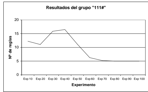
Figura 10: Evolución del número de reglas del grupo "111#" con el aumento de aleatoriedad en la generación del tablero.
