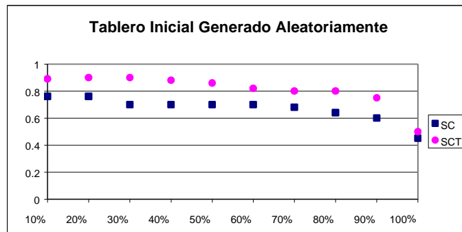
Figura 8: Tanto por ciento de partidas ganadas por el SCT y el SC clásico, promediando sobre 5 situaciones distintas, desde un tablero inicial generado aleatoriamente desde el 10% al 100%, frente a un contrincante 100% al azar.
