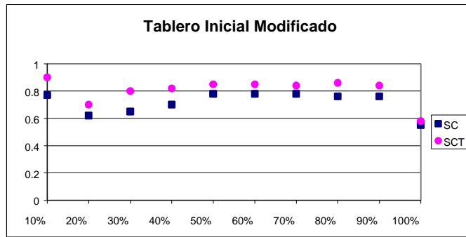
Figura 7: Tanto por ciento de partidas ganadas por el SCT y el SC clásico, promediando sobre 5 situaciones distintas, desde un tablero inicial modificado desde el 10% al 100%, frente a un contrincante 100% al azar.
