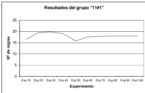
Figura 11: Evolución del número de reglas del grupo "11#1" con el aumento de aleatoriedad en la generación del tablero.
