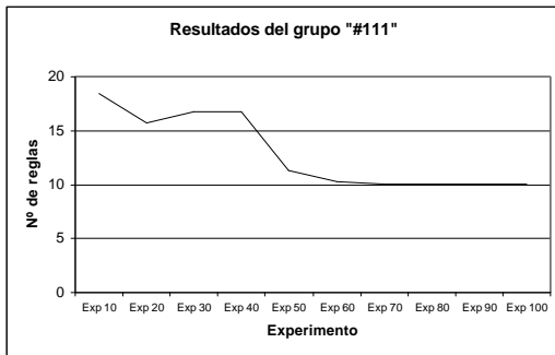
Figura 13: Evolución del número de reglas del grupo "#111" con el aumento de aleatoriedad en la generación del tablero.
