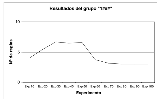
Figura 16: Evolución del número de reglas del grupo "1###" con el aumento de aleatoriedad en la generación del tablero.
