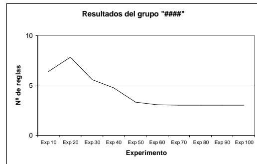
Figura 18: Evolución del número de reglas del grupo “####” con el aumento de aleatoriedad en la generación del tablero.
