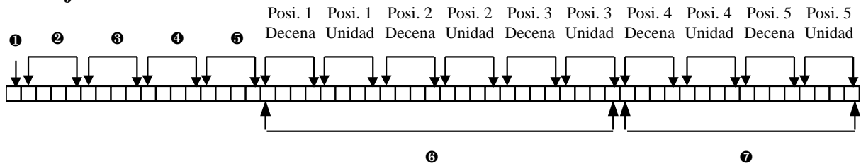
Figura 2: Mensaje de Entrada, y proceso de codificación de la información del tablero en la interfaz de entrada del SCT.
