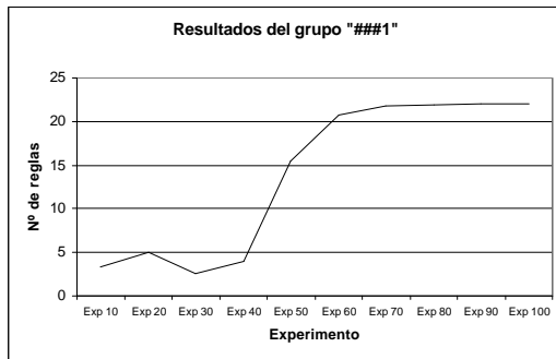
Figura 17: Evolución del número de reglas del grupo “##1” con el aumento de aleatoriedad en la generación del tablero.
