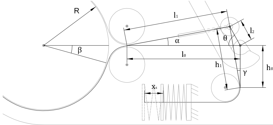
Figura 2. Esquema de funcionamiento del actuador de rigidez variable
