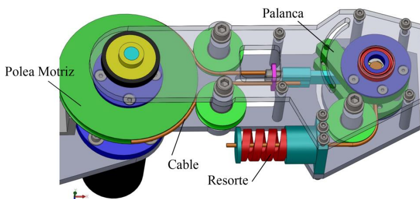
Figura 3. Diseño mecánico en 3D del MEVASTT
