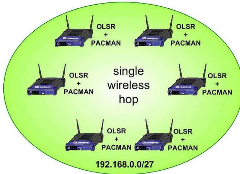
Fig. 3. Single-hop scenario.
