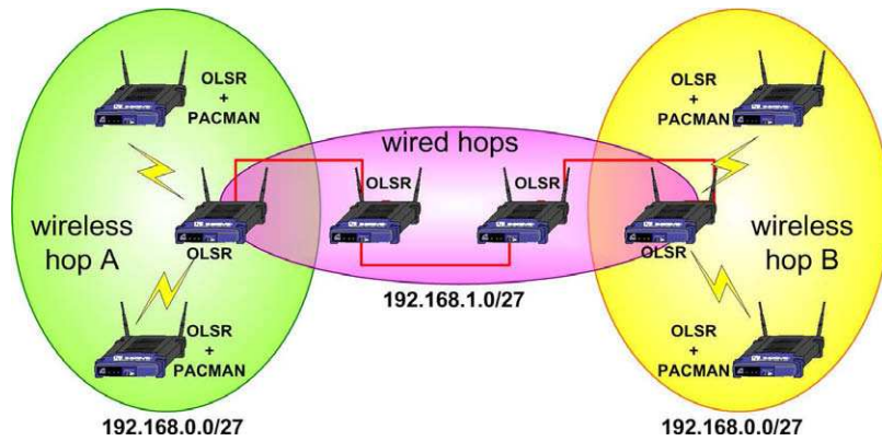
Fig. 10. Multiple-hop scenario.
