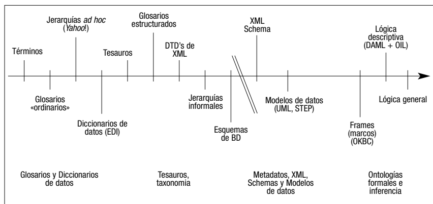
FIGURA 2. Tipos de ontologías según Gruninger y Uschold (2002)
