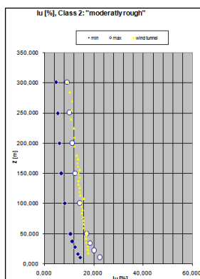
Figura 13 : Intensidad de la turbulencia en el aerogenerador 1
