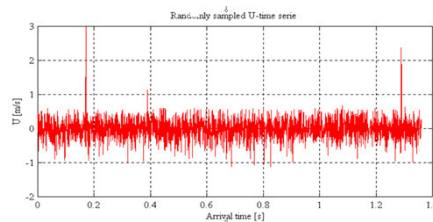
Figura 4 : Series temporales de la velocidad instantánea medida a partir de un flujo turbulento.
