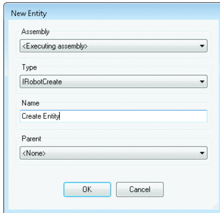
Figura 11. Inserción de una nueva entidad en el cuadro de diálogo New Entity
