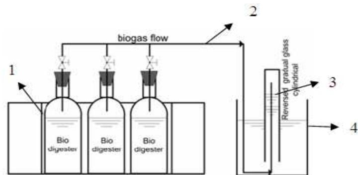
Gambar 1. Rangkaian alat produksi biogas (Budiono et al., 2010).
