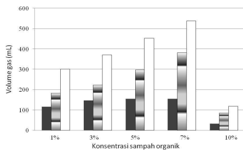
Gambar 3. Pengaruh konsentrasi sampah organik terhadap volume biogas (■: gas \text{CO}_2 , ▒: gas \text{CH}_4 , □: gas total)
