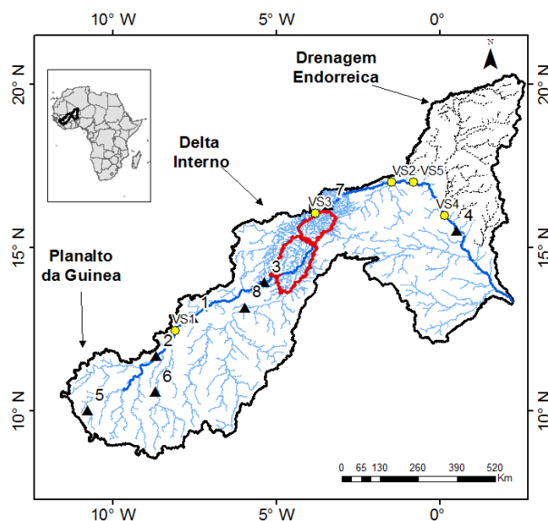
Figura 1 – Apresentação da bacia do Alto Rio Níger na África ocidental. Estão apresentadas as sete estações virtuais de altimetria espacial (círculos amarelos), as oito estações com observação utilizadas (triângulos pretos): Koulikoro (1), Banankoro (2), Ke-Macina (3), Ansongo (4), Faranah (5), Mandiana (6), Diré (7) e Douna (8). A rede de drenagem está apresentada em azul claro, rio principal em azul escuro, e drenagem endorreica que não contribui à bacia do Níger em preto.
