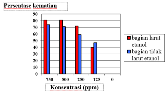
Gambar 3. Diagram hasil uji toksisitas bagian larut dan tidak larut etanol ekstrak metanol daun saga.
