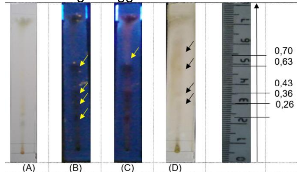
Gambar 1. Kromatogram hasil KLT ekstrak metanol daun saga deteksi dengan (A) sinar tampak, (B) sinar UV 254 , (C) sinar UV 366 (D) deteksi semprot serum (IV) sulfat.
