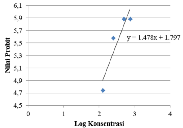
Gambar 4. Kurva regresi linier hasil uji toksisitas bagian larut etanol ekstrak metanol daun saga terhadap A. Salina
