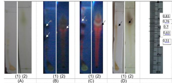
Gambar 2. Kromatogram hasil KLT partisi ekstrak metanol daun saga deteksi dengan (A) sinar tampak, (B) sinar UV 254 , (C) sinar UV 366 (D) deteksi semprot serum (IV) sulfat.
