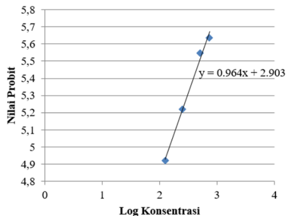
Gambar 5. Kurva regresi linier hasil uji toksisitas bagian tidak larut etanol ekstrak metanol daun saga terhadap A. salina
